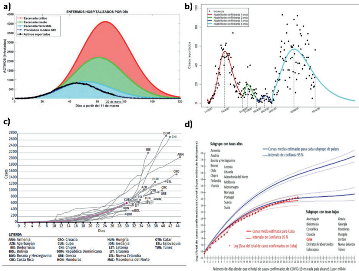
Fig. 2 A) Escenarios crítico (rojo), medio (verde) y favorable (azul) simulados con el modelo SIR con demografía en las primeras semanas de pandemia. En negro los datos reales, que abarcan el período desde el 11 de marzo hasta el 22 de mayo de 2020. B) Ajuste y predicción del modelo fenomenológico multionda implementado para los datos del período del 11 de marzo al 15 de octubre con predicción hasta diciembre. C) Curva de casos activos de COVID-19 en Cuba obtenida por el modelo de simulación con técnicas de inteligencia artificial a partir de los 20 países más similares a Cuba. D) Comparación de la tasa del total de casos confirmados en Cuba con respecto al crecimiento promedio de 2 subgrupos de países con características similares a Cuba.
