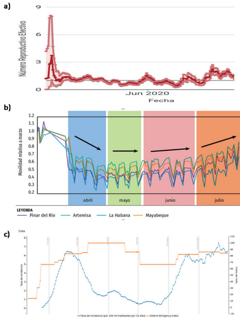
Fig. 4 Evolución del A) número reproductivo efectivo, B) índice de movilidad relativa a marzo de la población. Datos desde el 11 de marzo de 2020 al 31 de Julio de 2020, C) Tasa de incidencia de casos confirmados de COVID-19 e índice de rigor de Oxford en Cuba de 11 de marzo del 2020 a 30 de septiembre del 2020.
