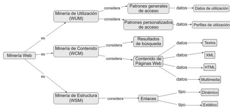
FIG. 1. Mapa conceptual de la clasificación minería Web, según Juan Carlos Dürsteler.
