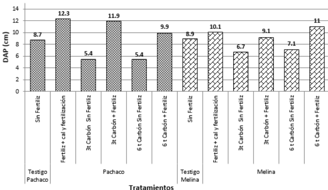
Fig. 3 - Promedio del Diámetro a la Altura del Pecho (DAP) por especie arbórea y nivel de fertilización a los dos años desde la plantación
