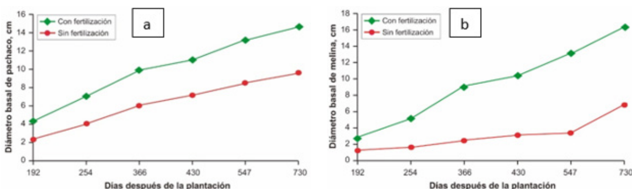
Fig. 2 - Evolución del Diámetro Basal de S. parahyba (a) y G. arborea (b) sin y con fertilización hasta los 730 días después de la plantación
