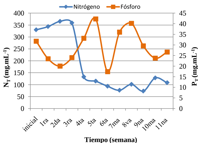
Figura 5. Contenido de nitrógeno total y fósforo total en el influente y efluente del proceso de biofiltración en serie
