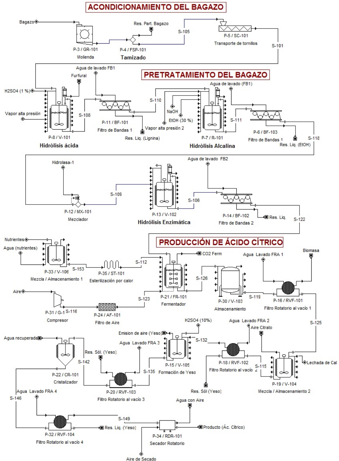
Figura 2. Esquema tecnológico para producción del Ácido Cítrico
