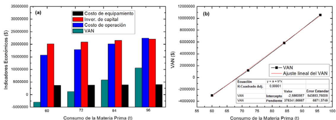
Figura 3. Indicadores económicos (a) Variación de los indicadores económicos respecto a la capacidad de la planta (b) Valor Actual Neto (VAN) vs consumo de materia prima y ecuación de ajuste
