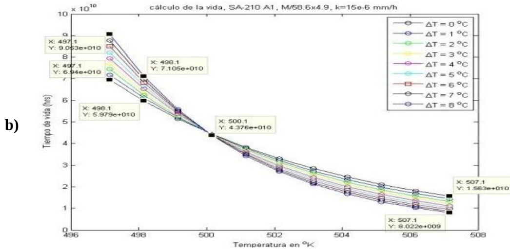
Figura 4. Vida por termofluencia en función de T °K y \Delta t °C para a) k=2,5 \times 10^{-6} mm/h, b) k=15 \times 10^{-6} mm/h para el acero SA-210 A1
