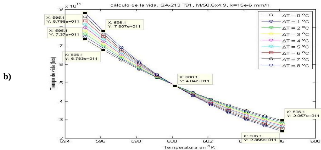
Figura 5. Vida por creep en función de T °K y \Delta t °C para a) k=2,5 \cdot 10^{-6} mm/h, b) k=15 \cdot 10^{-6} mm/h para el acero SA-213 T91
