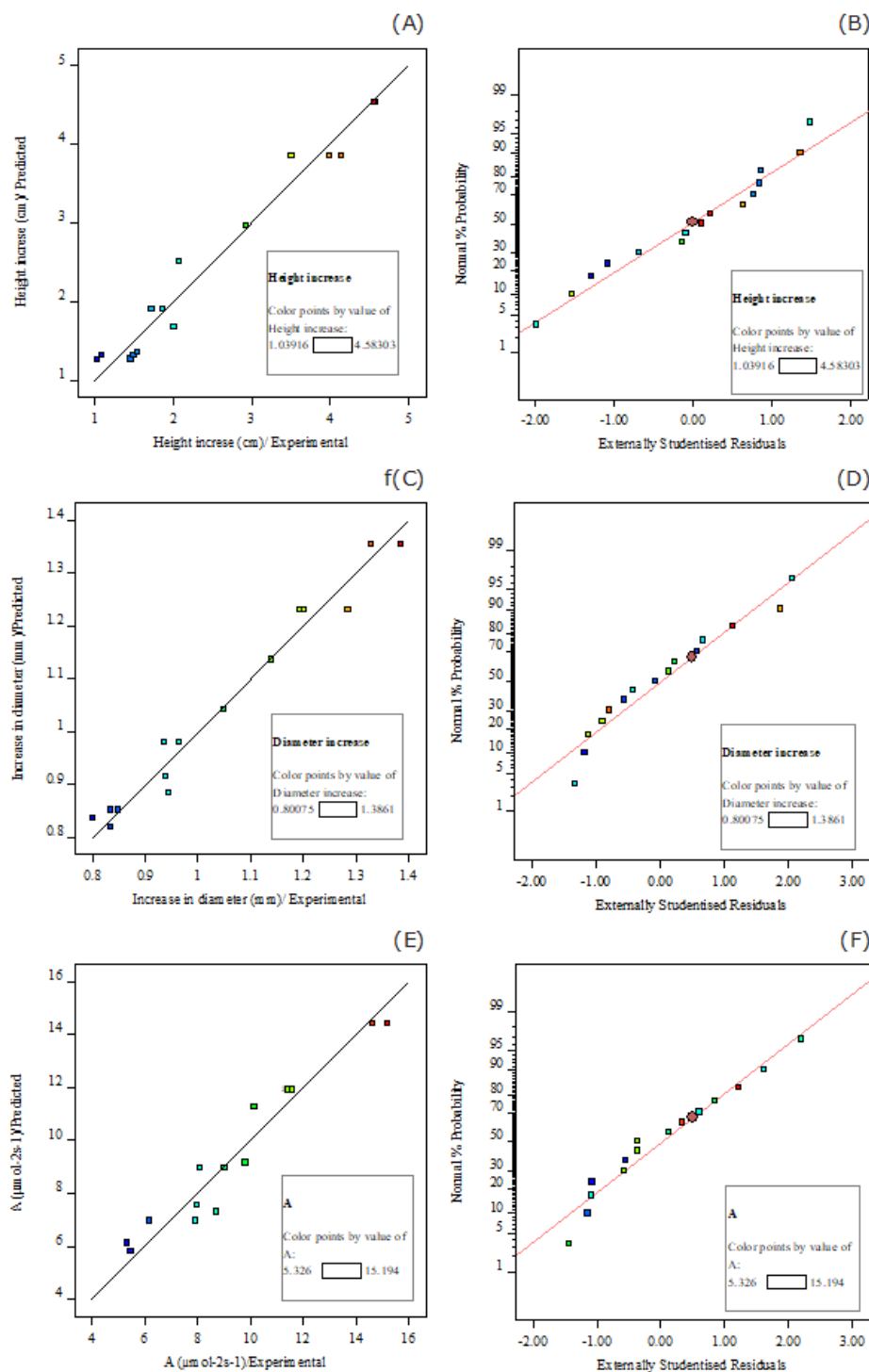
Figura 1. - Valores experimentales frente a los predichos para el diseño óptimo (personalizado): (A) aumento de la altura; (C) aumento del diámetro; (E) asimilación de CO 2 ; (B, D y F) distribución normal de los datos experimentales
