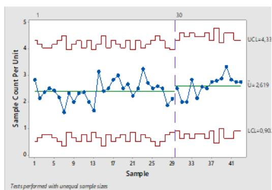
Figura 3. - Gráfico U de defectos para C3
