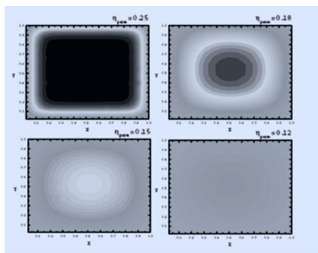
Figura 4 - Distribución de la humedad en la sección transversal de la pieza con el avance del secado para un contenido de humedad en la frontera del 10 %
