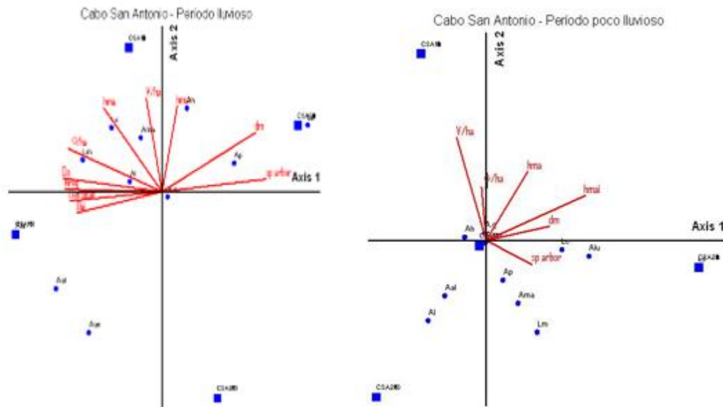
Figura 5. - Diagrama de ordenación de análisis de correspondencia realizado con la densidad especies de lagartos y las variables de vegetación en el sector Cabo de San Antonio
