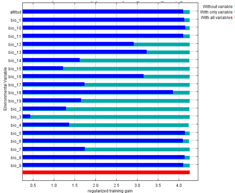
Figura 4. - Contribución de las variables ambientales al modelo de distribución potencial actual de Magnolia cubensis subsp. cubensis en el oriente de Cuba
