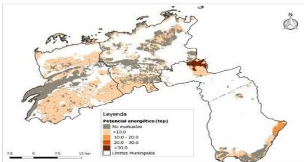
Figura 9. - Potencial energético por rodal
