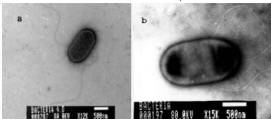
Figura 2. Microfotografía al microscopio electrónico de transmisión a) Aislado T2 de Gluconacetobacter diazotrophicus b) Aislado 9C de Pantoea sp. ambos microorganismos tienen forma de bacilo
