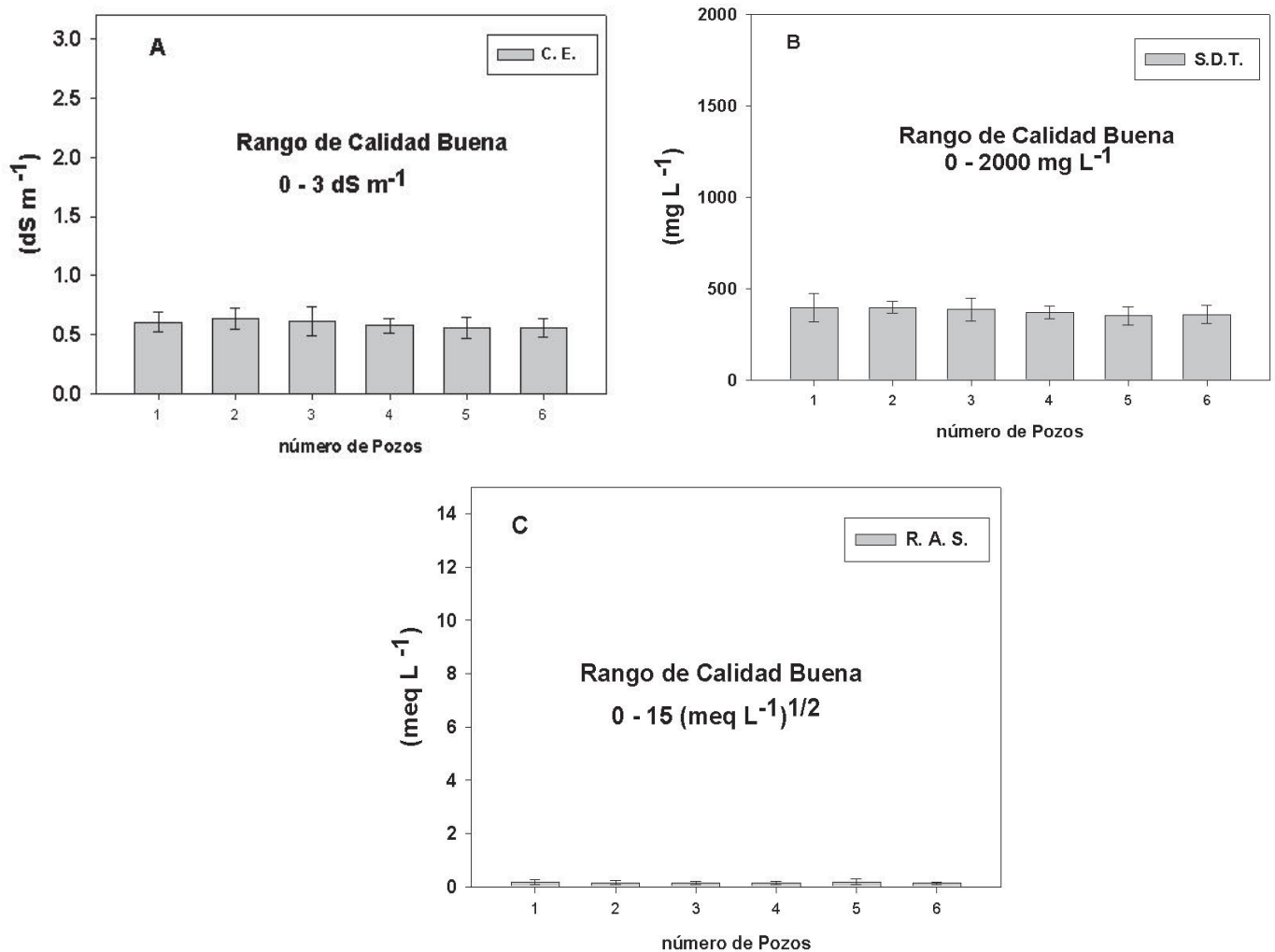
Figura 2. Variación de los valores de conductividad eléctrica (A), sales disueltas totales (B) y relación de absorción de sodio (C) en los seis pozos de explotación alta, durante los 14 meses de evaluación
