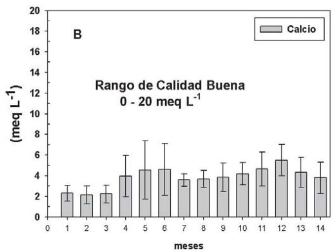
Figura 5. Comportamiento mensual de los valores de pH (A) y calcio (B) en cada uno de los seis pozos de explotación alta
