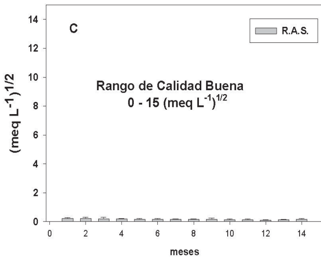
Figura 4. Comportamiento mensual de los valores de conductividad eléctrica (A), sales disueltas totales (B) y relación de absorción de sodio (C) en cada uno de los seis pozos de explotación alta
