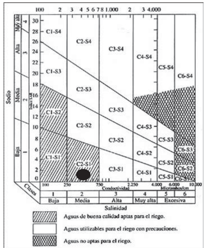
Figura 1. Normas de Riverside para evaluar la calidad de las aguas de riego (U.S. Soil Salinity Laboratory)
