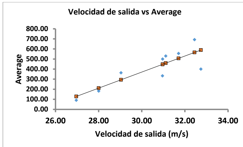
Fig. 5. - Average vs velocidad de salida
