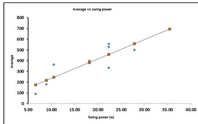
Fig. 6. - Average vs potencia del swing
