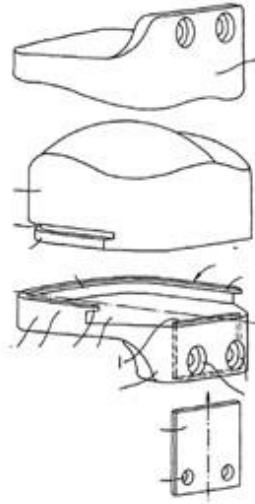
Fig. 10: Intervertebral Prosthesis With a Limit Stop Plate. United States. Patente n.º US 8 062 370 B2.
