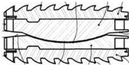
Fig. 12: Prothese de disque pour vertebres cervicales. Republique française. Patente n.º FR 2 951 930 - A1.
