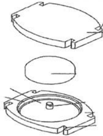
Fig. 15: Prótesis de disco intervertebral. España. Patente n.º ES 2 367 685 T3.
