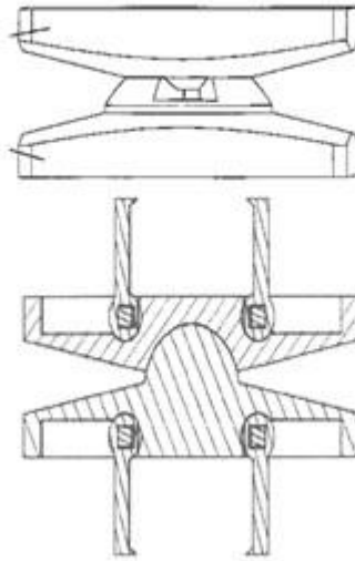
Fig. 11: Inter-vertebral disc prosthesis. United States. Patente n.º US 8 303 660 B1.
