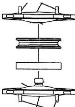
Fig. 8: Prótesis de disco intervertebral de aplicación universal. España. Patente n.º ES 2 331 007.
