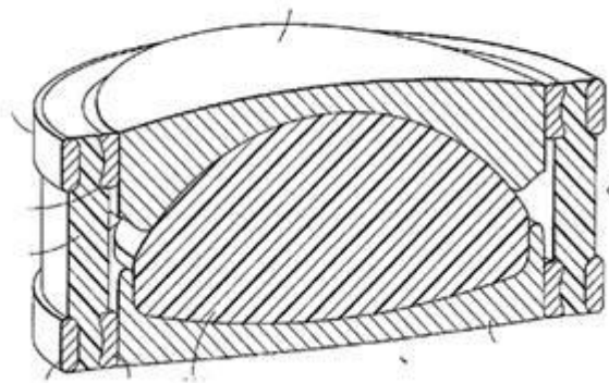
Fig. 3: Artificial intervertebral disc. United States. Patente n.º US 8 388 685 B2.
