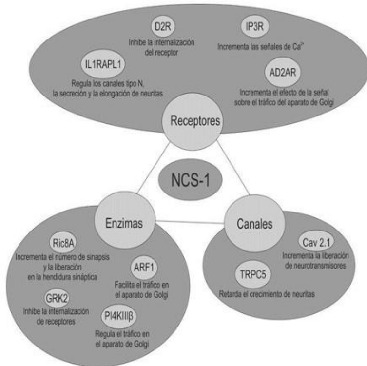
Fig. 2. Efectos funcionales de las interacciones entre NCS-1 y proteínas blanco. En el esquema se puede observar un resumen de las interacciones de NCS-1 con proteínas que tiene un efecto funcional demostrado en la fisiología neuronal. IP3R: Receptor de inositol trifosfato. D2R: receptor D2 dopaminérgico. GRK2: Kinasa acoplada a proteínas G-2. TRPC5: Transient
