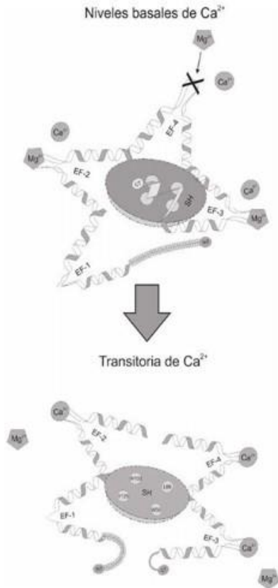
Fig. 1. Representación esquemática de la interacción de NCS-1 con Ca^{2+} . A niveles basales de Ca^{2+} (parte superior de la figura), EF-2 y 3 se encuentran unidos a Mg^{2+} ; en este estado el extremo carboxilterminal de la proteína, ubicado cerca de EF-3, se repliega para cubrir los aminoácidos que corresponden a los sitios de unión de la SH utilizados por la NCS-1 para acoplarse a sus proteínas blanco, también se observa la cadena miristoil unida al extremo aminoterminal, la cual es clave para el acople a la membrana plasmática. Cuando ocurre una elevación de la concentración de Ca^{2+} , éste logra desplazar los iones de Mg^{2+} y se une a las EF-2, EF-3 y a EF-4 ocasionando un cambio conformacional desplazando el segmento carboxilterminal y exponiendo los sitios de unión en la SH para permitir que la NCS-1 logre acoplarse a sus proteínas blanco.
