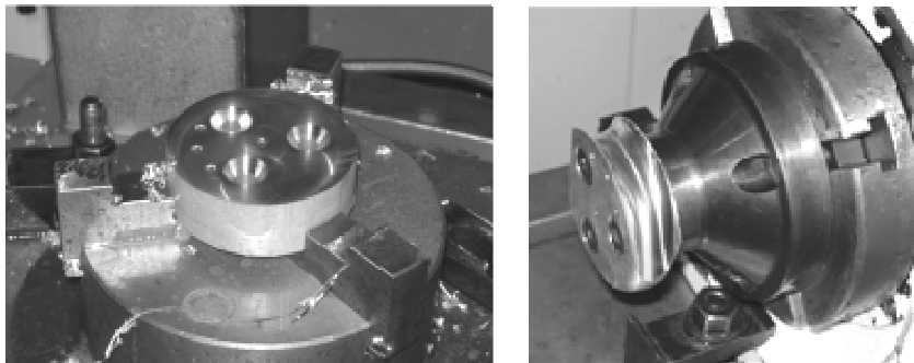
Fig.8. A la izquierda proceso de preparación de la materia prima para el montaje. A la derecha parte final obtenida
