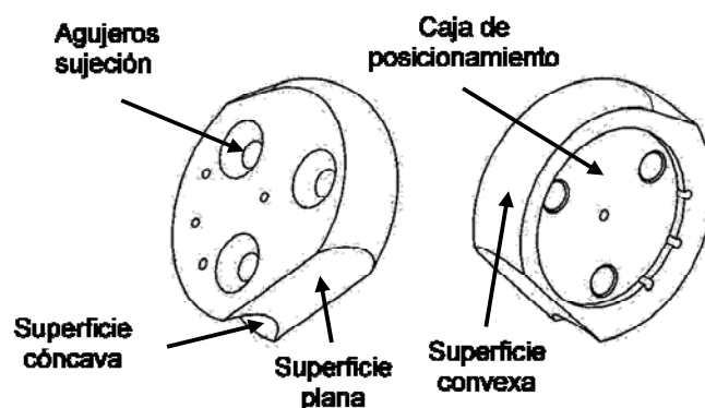
Fig. 5. Pieza experimental e identificación de sus características funcionales
