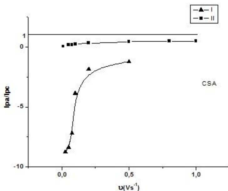
Figura 7. Gráfico de I_{pa}/I_{pc} versus velocidad de barrido, electrodo modificado pirrol/CSA (I Fe 10^{-3} mol L ^{-1} II Fe 10^{-4} mol L ^{-1} )
