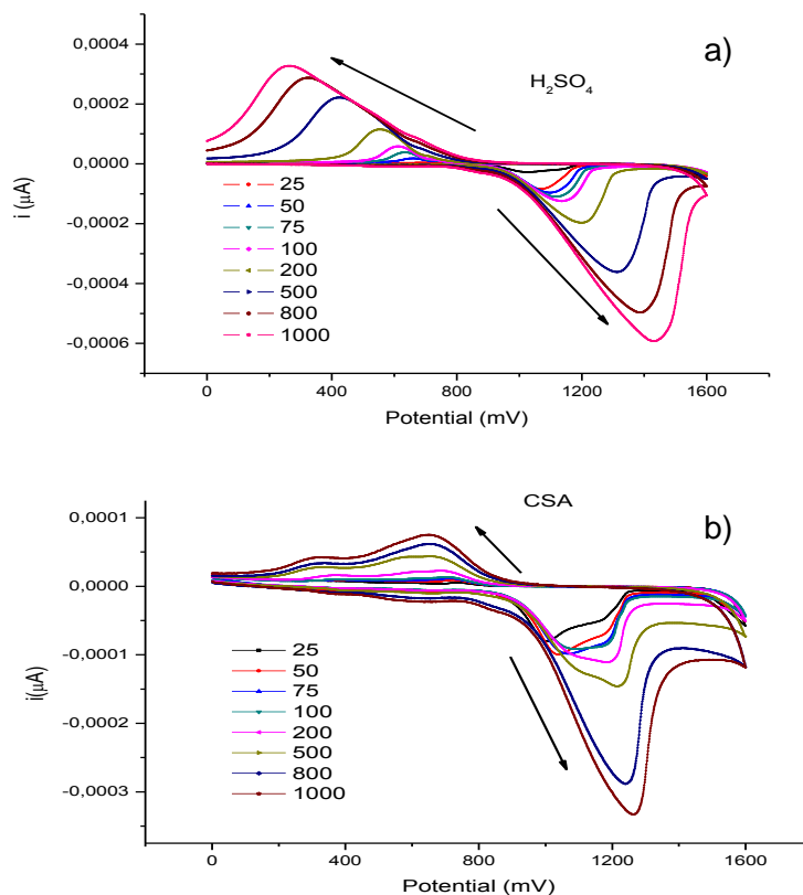
Figura 4. Perfil voltamétrico a diferentes velocidad de barrido para a) sistema pirrol/ \text{H}_2\text{SO}_4 y b) sistema pirrol/CSA, solución de \text{Fe}(\text{CN})_6^{3-/4} 10^{-3} \text{ mol.L}^{-1}
