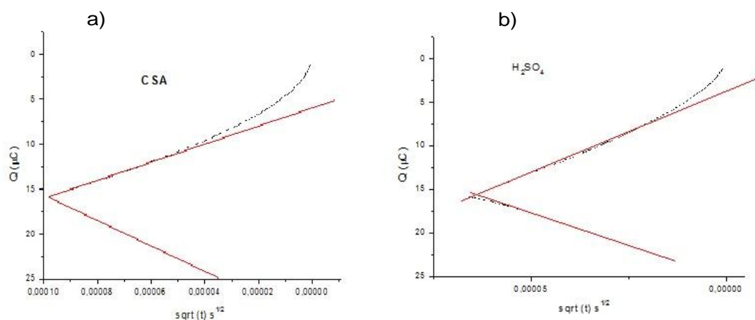
Figura 2. Diagramas de Anson: a) pirrol/CSA y b) pirrol/H 2 SO 4
