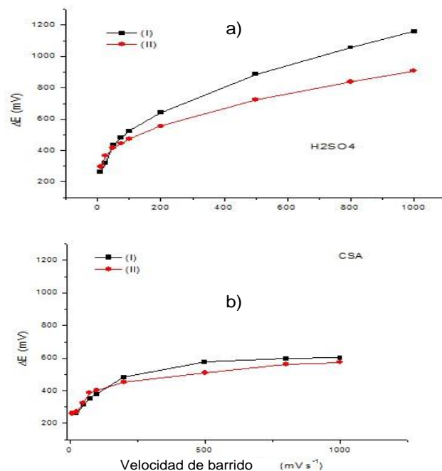
Figura 5. Gráficos de \Delta E versus velocidad de barrido, (I Fe 10^{-3} mol L ^{-1} , II Fe 10^{-4} mol L ^{-1} ) a) sistema pirrol/H 2 SO 4 y b) sistema pirrol/CSA
