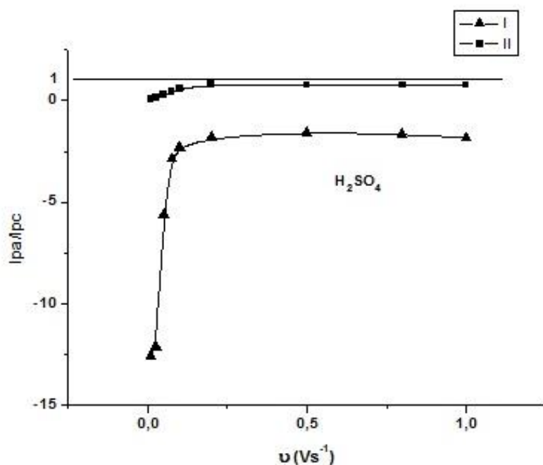
Figura 6. Gráficos de I_{pa}/I_{pc} versus velocidad de barrido, electrodo modificado pirrol/H 2 SO 4 , (I Fe 10^{-3} mol L ^{-1} , I Fe 10^{-4} mol L ^{-1} )
