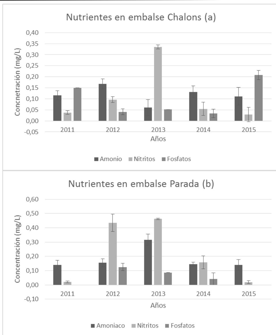
Fig. 4. Concentración de nutrientes en los embalses Chalons (a) y Parada (b)
