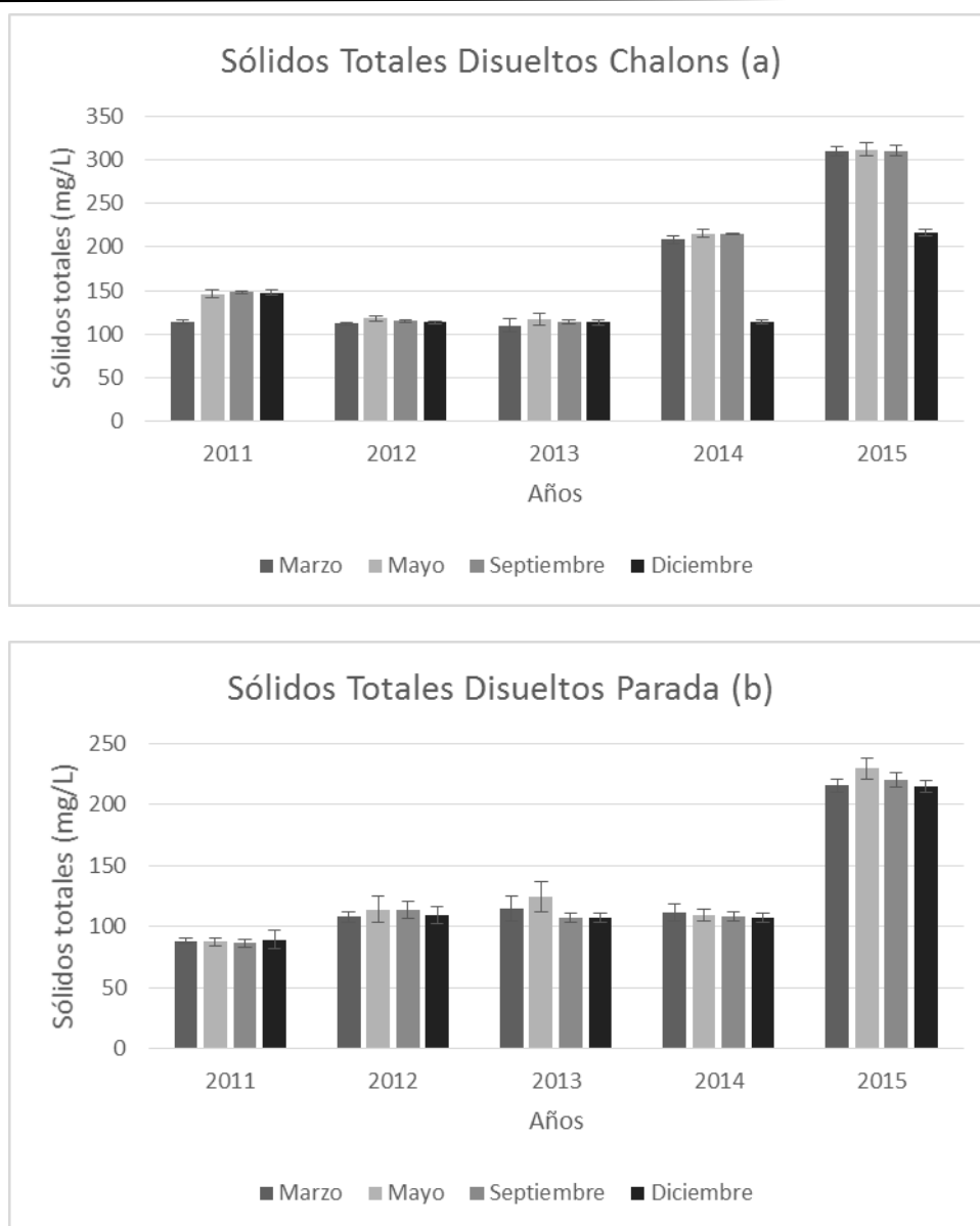
Fig. 3. Sólidos Totales Disueltos de los embalses Chalons(a) y Parada (b) período 2011-2015
