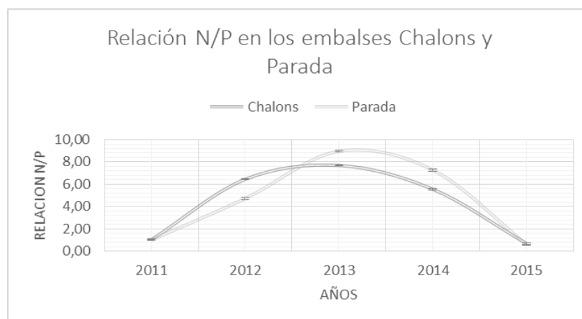
Fig. 5. Relación N/P en los embalses Chalons y Parada
