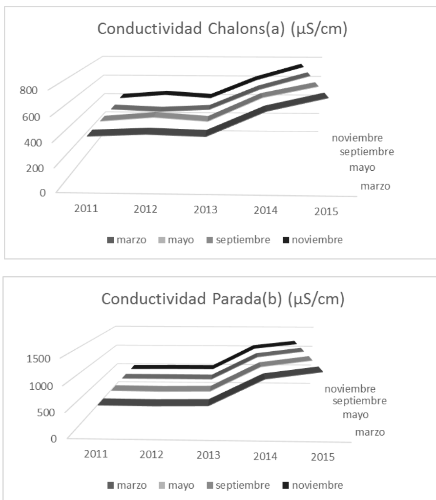
Fig. 1. Conductividad en los embalses Chalons (a) y Parada (b) en el período 2011-2015
