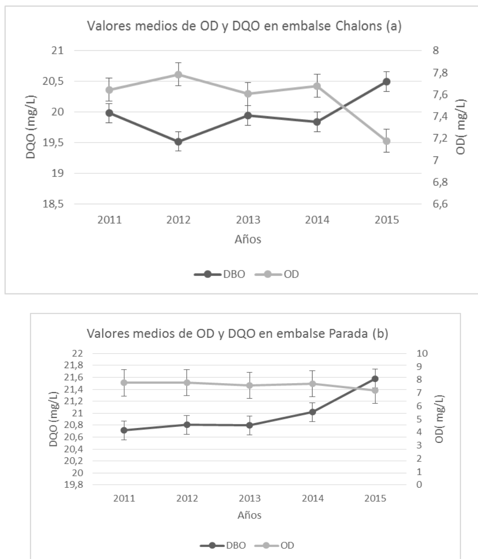
Fig. 6. Niveles de Oxígeno Disuelto (OD) y Demanda Química de Oxígeno (DQO) en los embalses Chalons (a) y Parada (b)
