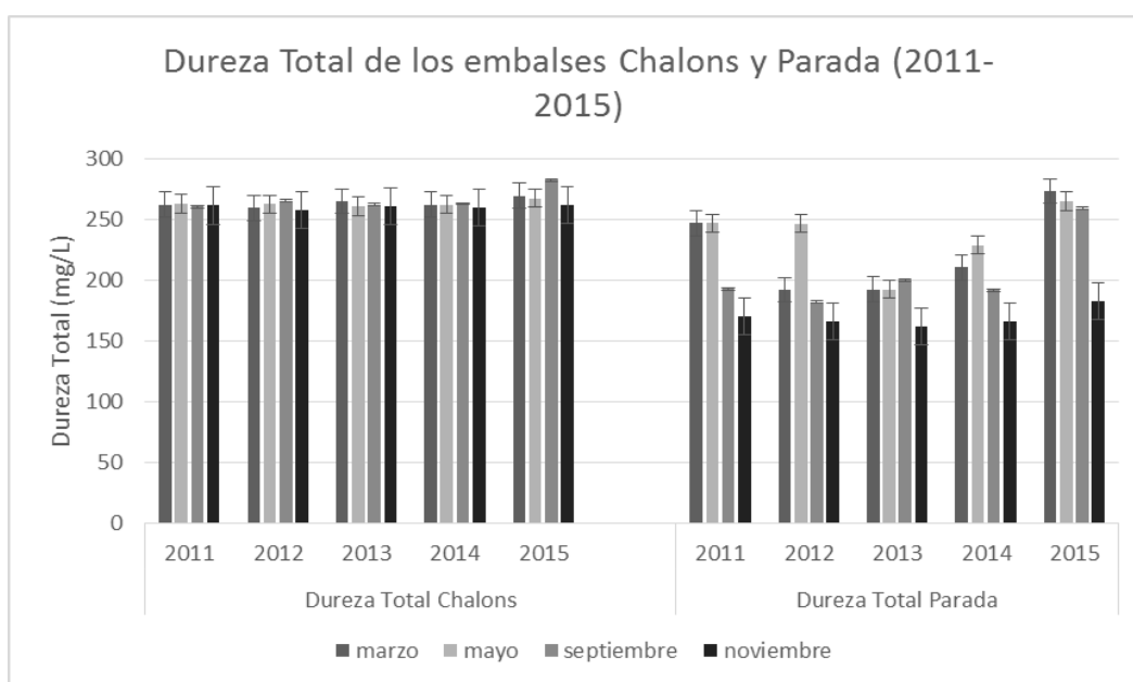
Fig. 2. Variación de la dureza total en los embalses Chalons y Parada (2011-2015)
