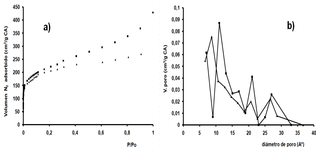
Fig. 1 Adsorción de N 2 a 77 K: CA/ML (▲) CA/NE (■) a) Isotherma de adsorción de N 2 b) Distribución de poros
