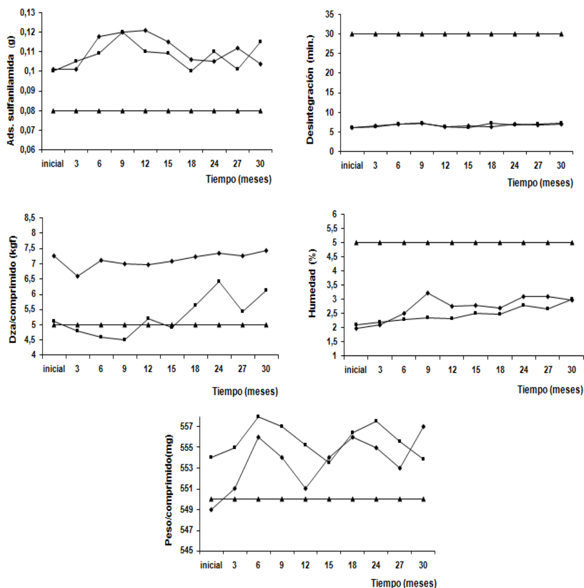
Fig. 3 Estabilidad vida de estante: CA/ML (♦) CA/NE (■) Especificaciones (▲)
