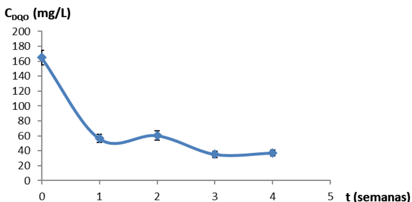
Fig. 2. Comportamiento de la remoción de la DQO
