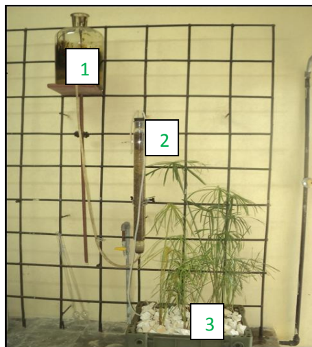
Fig. 1. Sistema experimental utilizado, compuesto por tanque estabilizador (1), columna de absorción (2) y humedal construido (3)
