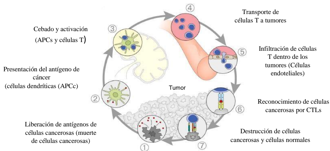
Fig. 1 - Representación del ciclo de inmunidad contra el cáncer, que ilustra la respuesta inmune a un tumor (13) , (figura modificada con autorización de los autores)
