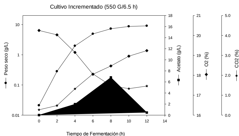
Fig. 4A - Influencia del campo magnético, en el crecimiento celular y la concentración de metabolitos del proceso productivo de la proteína recombinante Gp-41, utilizando cultivo incrementado
