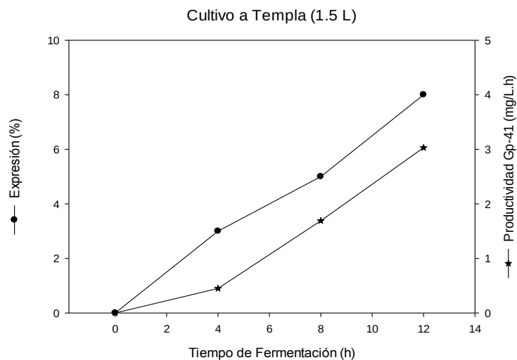
Fig. 2B - Nivel de expresión y productividad del proceso de obtención de la proteína recombinante Gp-41 a nivel de 1,5 L, utilizando cultivo a Templa
