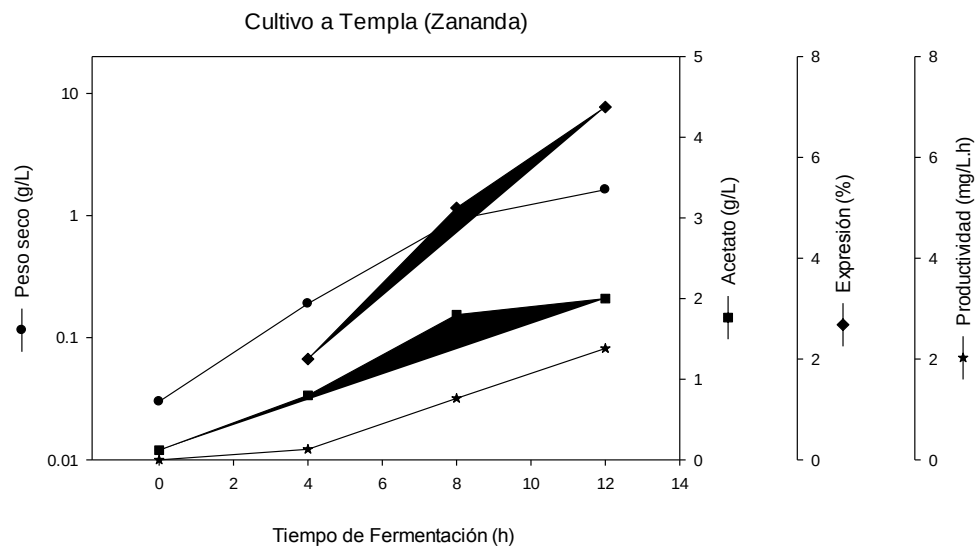
Fig. 1 - Evaluación del proceso productivo de la proteína recombinante Gp-41, utilizando cultivo a Templa, en zaranda
