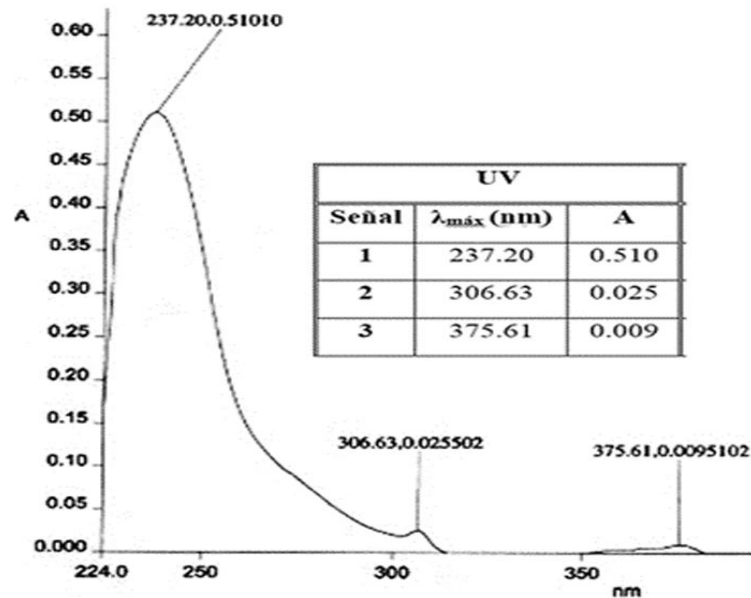
Fig. 1 - Perfil del espectro de absorción UV-Vis del AE del rizoma de C. longa L
