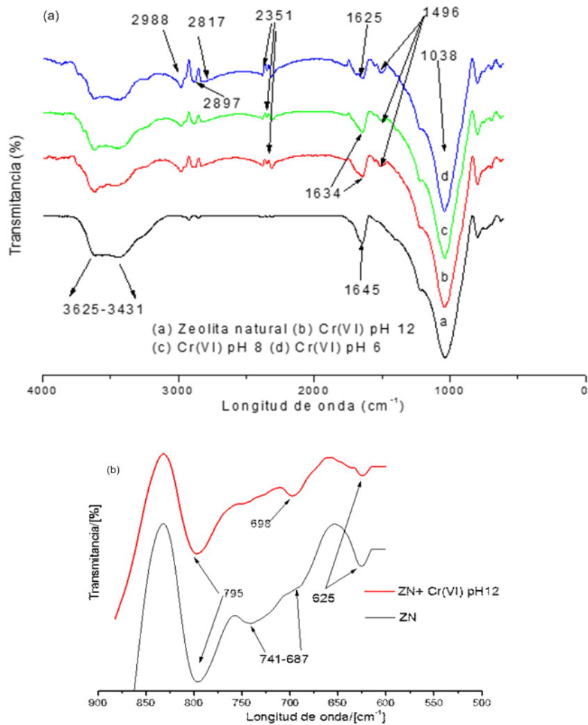
Fig. 2- (a) Espectro FT-IR de la ZN natural y tratada con disolución de \text{CrO}_4^{2-} [Cr (VI)] de 4,69 mg/L a diferentes valores de pH. (b) Imagen ampliada de una porción de (a).
