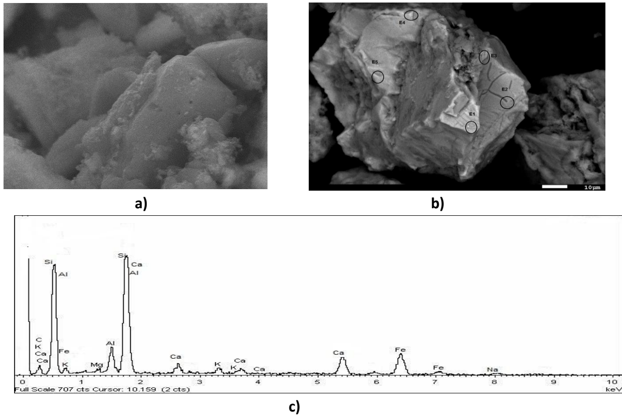
Fig. 4 - Micrografías de la zeolita natural “x 20μm” (a) y la zeolita tratada “x 10μm” (b) con disolución de \text{CrO}_4^{2-} = 0,465 mg/L y pH 12,3; así como el EDX (c) de la zeolita natural
