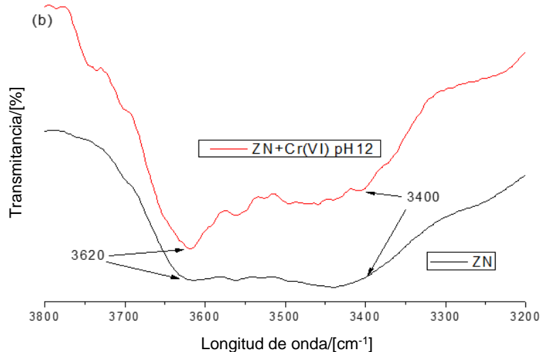
Fig. 3 - Espectros FT-IR de la ZN tratada con disolución de \text{CrO}_4^{2-} [Cr (VI)] de 4,69 mg/L a diferentes valores de pH
