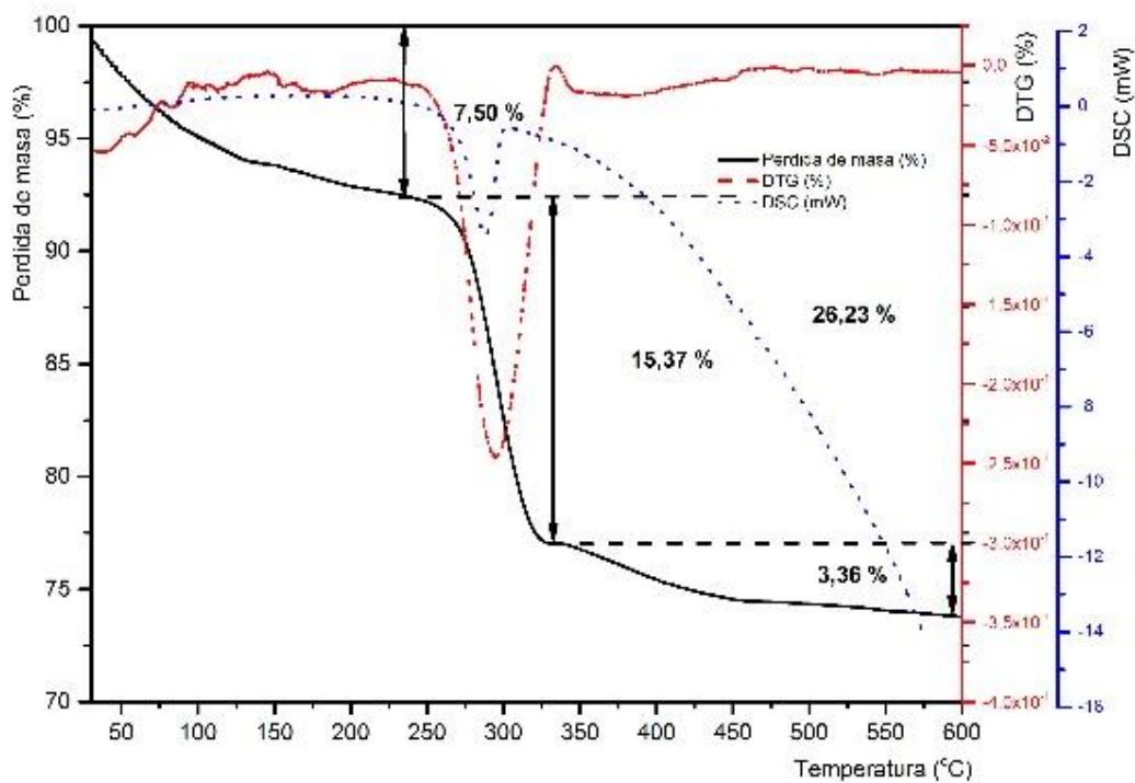
Fig. 3- Curvas TG y DSC del hidróxido de níquel (II) obtenido con licor industrial (muestra B)
