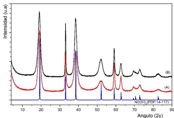
Fig. 1- Difractogramas de las muestras de hidróxido de níquel obtenidas a partir del sulfato de níquel del (A) licor sintético y del (B) licor industrial
