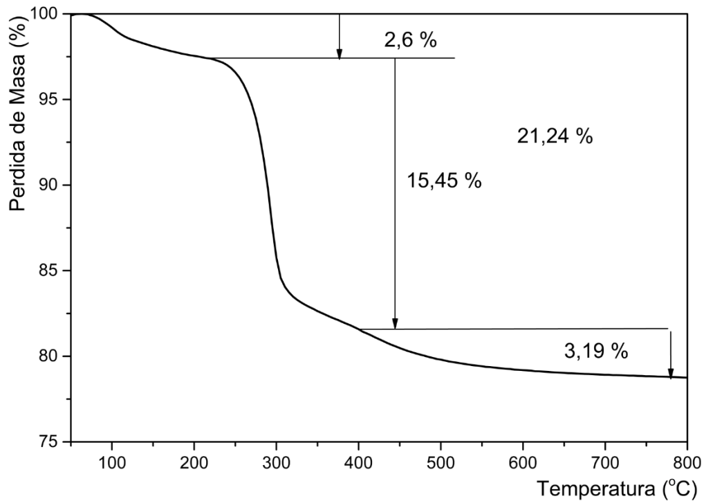
Fig. 2- Curvas TG del hidróxido de níquel (II) de referencia (muestra A)
