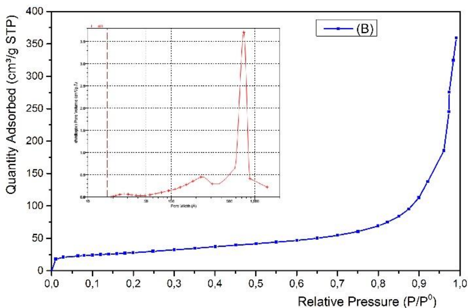
Fig. 6- Isothermas de adsorción de nitrógeno de los hidróxidos de níquel, se insertan las curvas de distribución de poros. A: hidróxido de referencia. B: hidróxido obtenido con licor industrial
