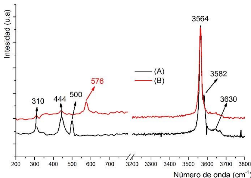
Fig. 5- Espectro Raman del Ni(OH) 2 obtenido a partir de licor sintético (A) y licores industriales (B)
