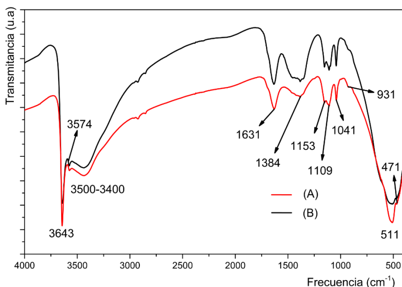
Fig. 4- Espectro FTIR del Ni(OH) 2 obtenido a partir de (A) licores reactivos y (B) licores industriales
