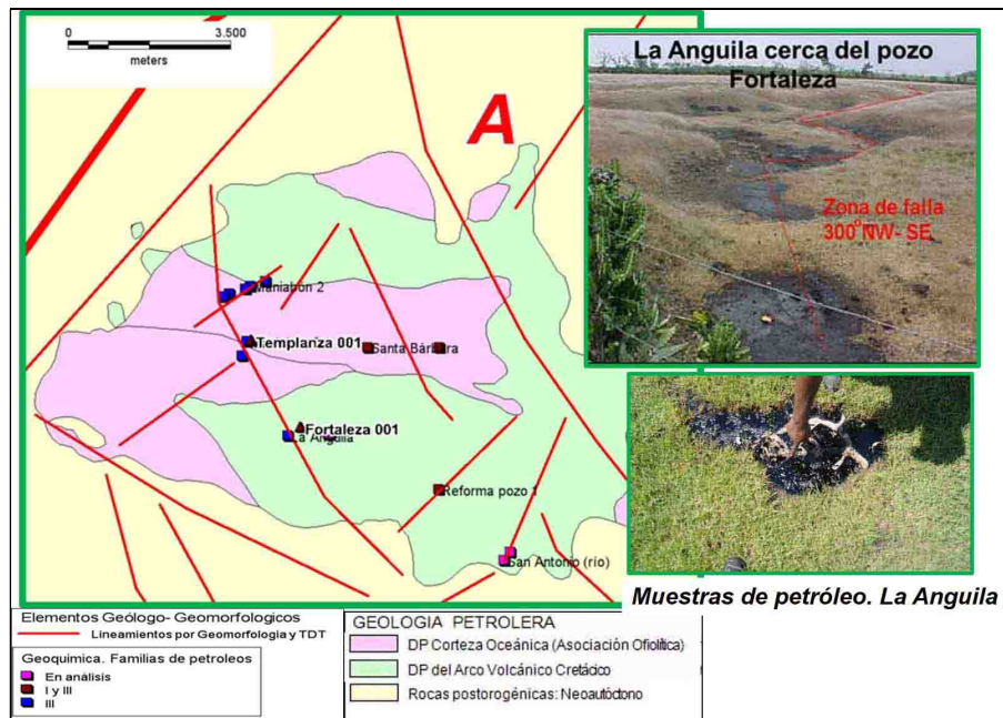
Figura 3. Esquema morfoestructural integrado con la geología de superficie (izquierda), donde se evidencia la relación espacial de los sistemas de lineamientos con las manifestaciones superficiales de petróleo. Puntos dentro del área que demuestran la ocurrencia de abundantes emanaciones activas (derecha abajo). Nótese la relación de la zona de falla con las manifestaciones de petróleo (derecha arriba).
