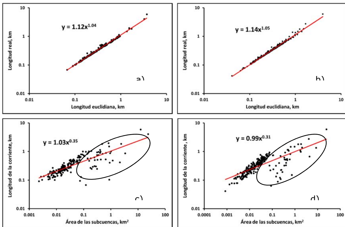
Figura 4. Determinación de la dimensión fractal promedio de la corriente para los ríos San Cristóbal y Santa Cruz a partir de las pendientes de las rectas ajustadas. a) y b) según Takayasu (1990); c) y d) según Mandelbrot (1983). Las elipses encierran los ríos que se alejan de la nube principal, mayormente de orden dos en adelante.
