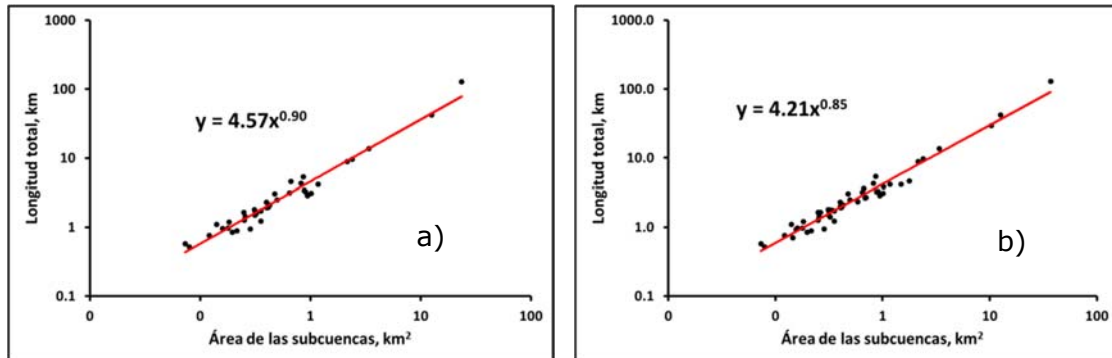
Figura 5. Gráficos para la estimación del parámetro \epsilon , empleado en cálculo de la dimensión fractal de la red: a) río San Cristóbal, b) río Santa Cruz. El eje de las ordenadas representa la longitud total de todas las corrientes que caen dentro de una subcuenca.
