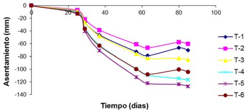
Figura 5. Asentamiento de los puntos de control.
