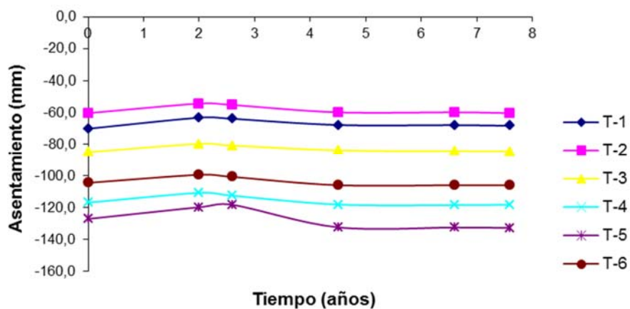
Figura 7. Asentamientos durante el proceso de explotación.
