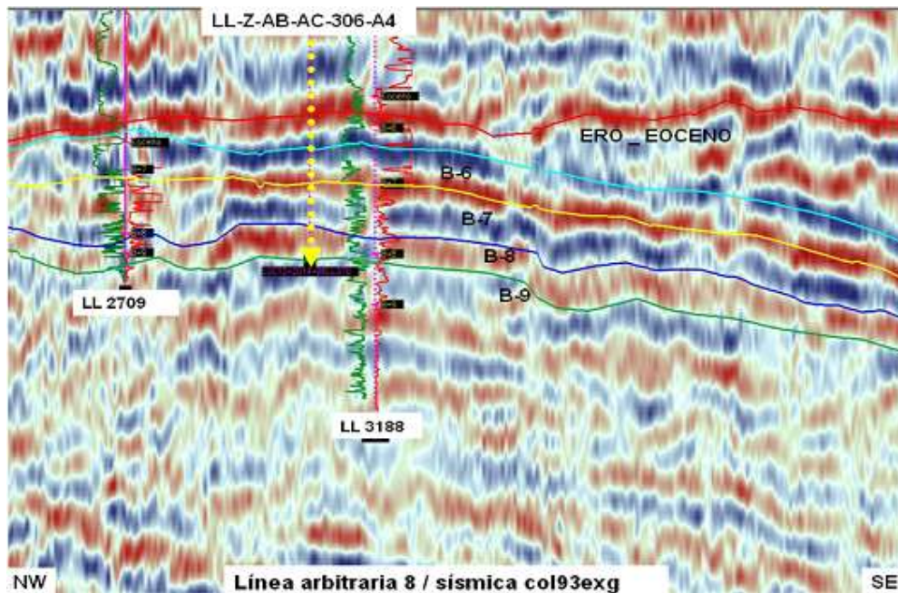
Figura 4. Línea sísmica de dirección NO-SE.
