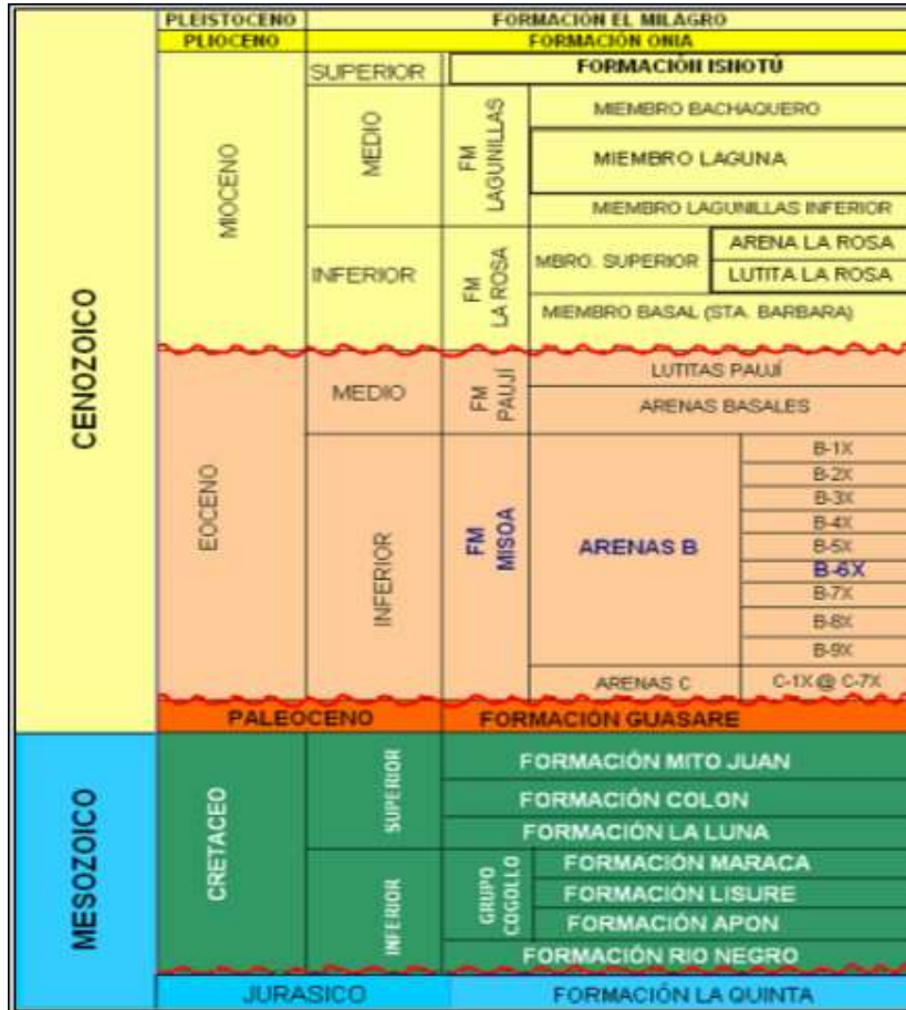
Figura 2. Columna estratigráfica del campo Tía Juana Lago.
