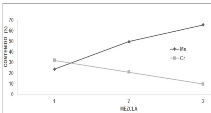
Figura 3. Contenidos de Mn y Cr en las ferroaleaciones obtenidas.
