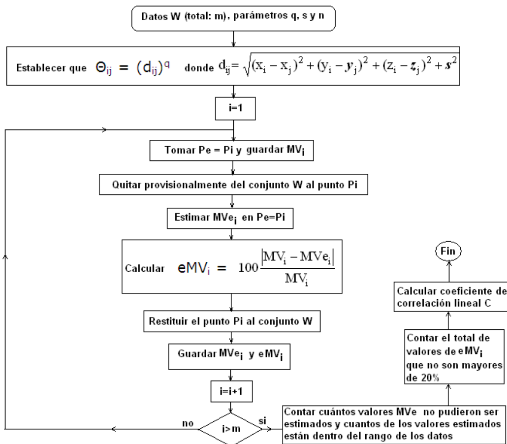
Figura 4. Algoritmo del procedimiento de validación cruzada.
