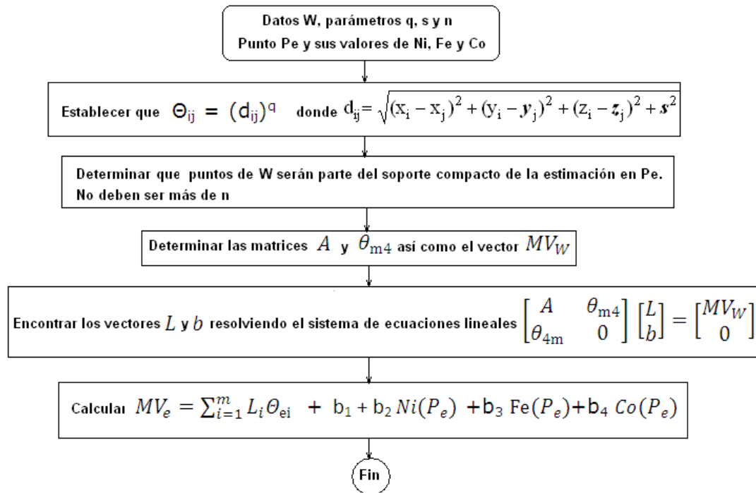
Figura 1. Algoritmo del estimador puntual UPD propuesto.
