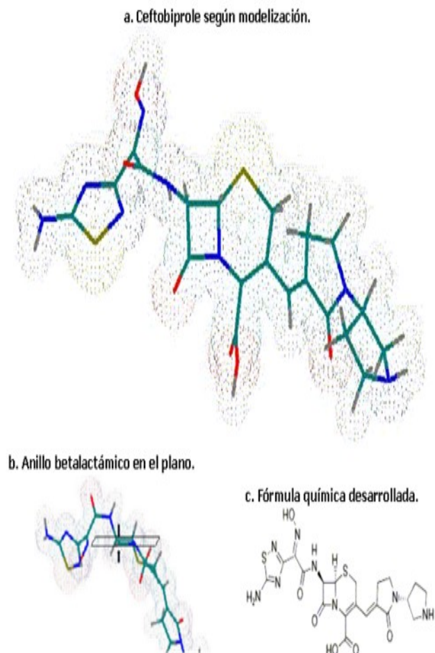
Figura 3. Cefotaxime: a. Estructura tridimensional optimizada con cálculos semiempíricos PM3; b. Vista con el anillo betalactámico en el plano horizontal, las flechas señalan el carbono carbonílico (C8) y c. Fórmula química desarrollada.
