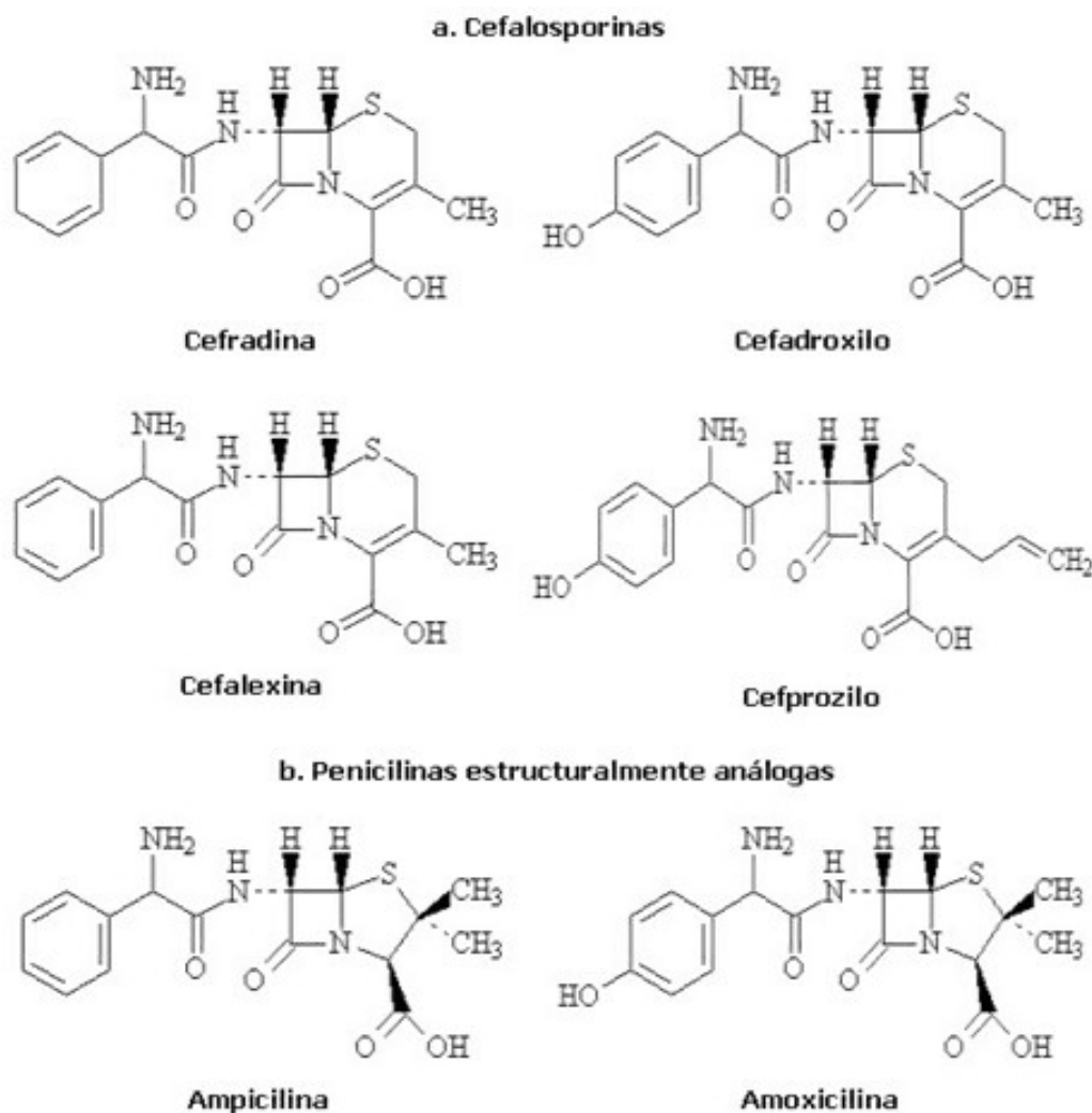
Figura 1. Estructuras químicas de: a. Cefalosporinas modeladas y b. Penicilinas estructuralmente análogas, estudiadas en un trabajo precedente. (44)
