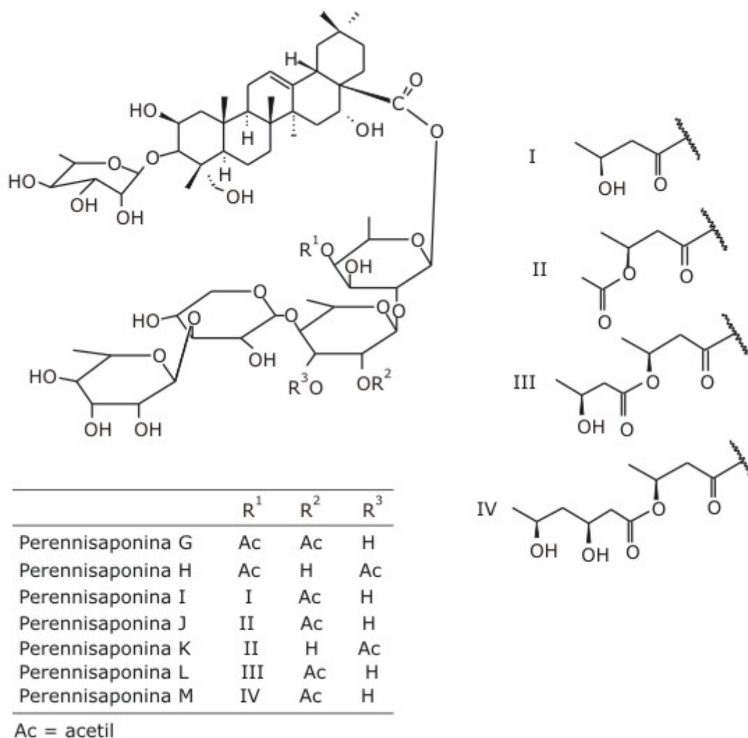
Fig. 3. Perennisaponinas G, H, I, J, K, L e M. Fonte: Morikawa et al., 21 2010.
