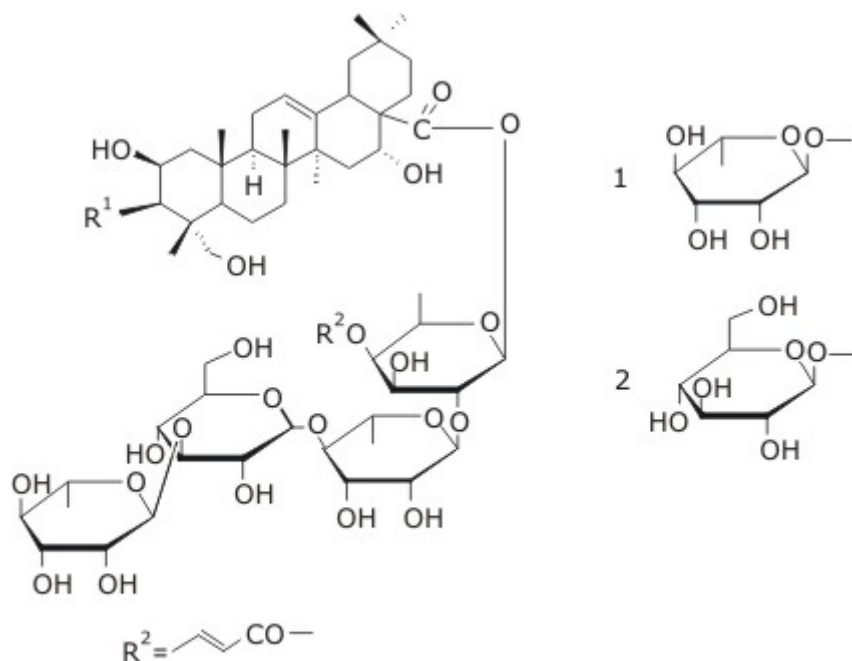
Fig. 2. Belisaponinas BA1(1) e BA2 (2). Fonte: Schöpke et al.,1991. 20
