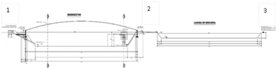
1: antes de entrar al digestor, 2: después de salir del digestor, 3: salida del lago de estabilización. Figura 1. Puntos de muestreo para el análisis de los residuales.
