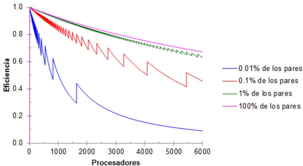
Figura 8. Comportamiento estimado de la eficiencia en el cálculo paralelo del perfil físico-químico par a par de secuencias
