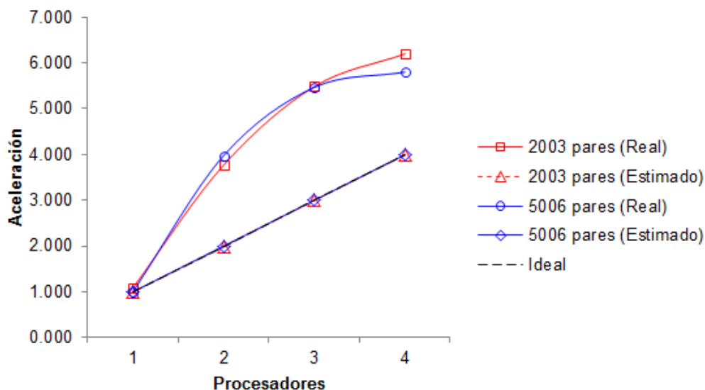
Figura 9. Comportamiento experimental de la aceleración en el cálculo paralelo de los alineamientos par a par de secuencias
