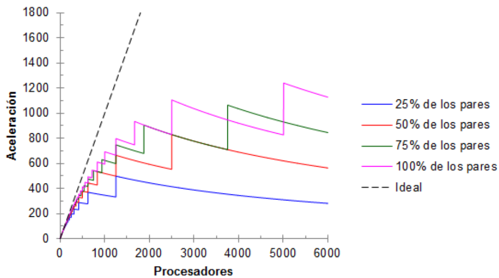
Figura 5. Comportamiento estimado de la aceleración en el cálculo paralelo de los alineamientos par a par de secuencias.
