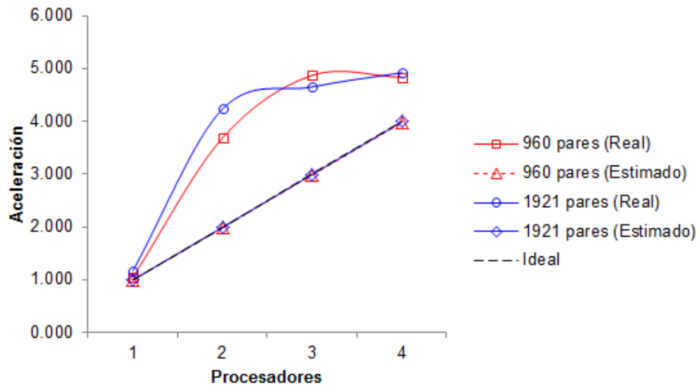
Figura 11. Comportamiento experimental de la aceleración en el cálculo paralelo del perfil físico-químico par a par de secuencias de proteínas.
