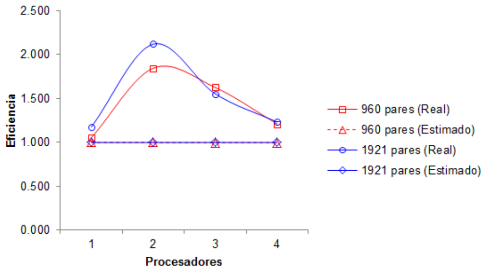
Figura 12. Comportamiento experimental de la eficiencia en el cálculo paralelo del perfil físico-químico par a par de secuencias de proteínas
