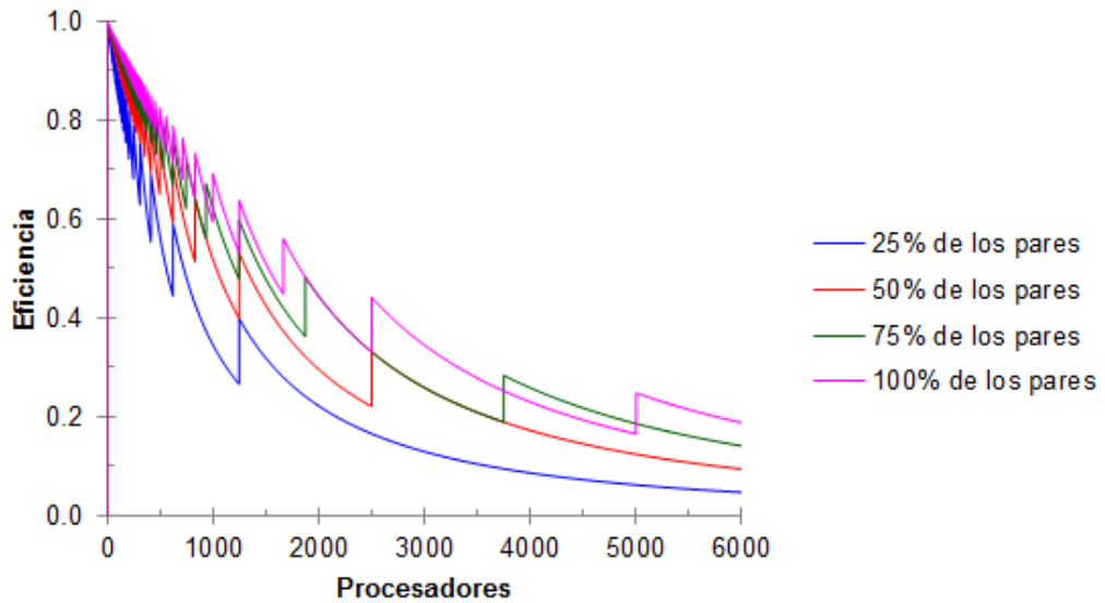
Figura 6. Comportamiento estimado de la eficiencia en el cálculo paralelo de los alineamientos par a par de secuencias
