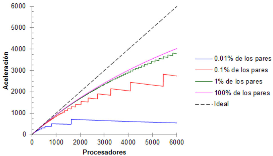
Figura 7. Comportamiento estimado de la aceleración en el cálculo paralelo del perfil físico-químico par a par de secuencias
