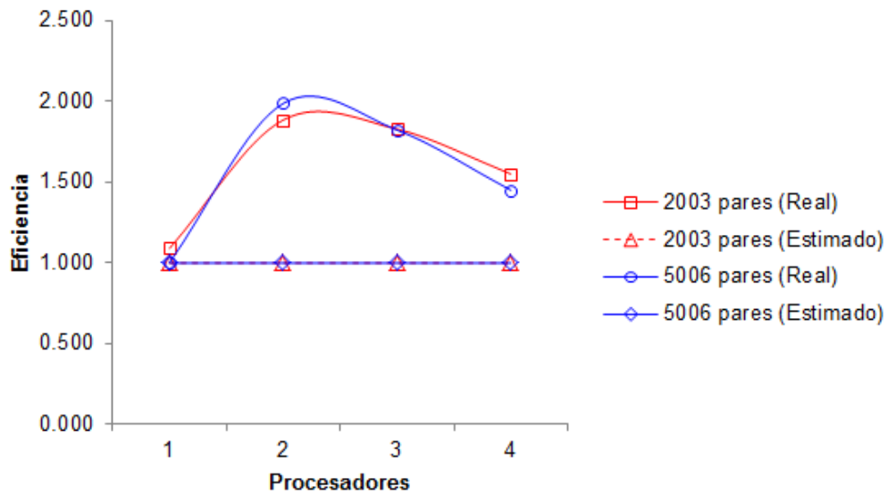
Figura 10. Comportamiento experimental de la eficiencia en el cálculo paralelo de los alineamientos par a par de secuencias
