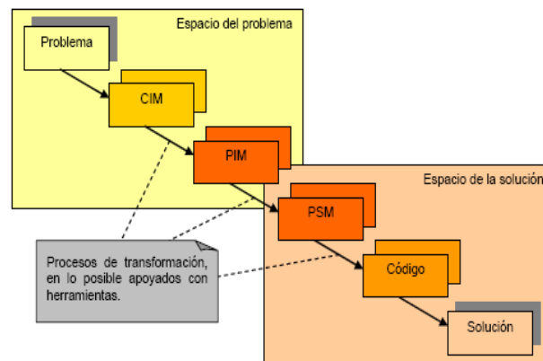
Fig. 1- Proceso de desarrollo con MDA. (Peña-Moreno 2011)
