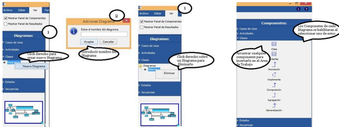
Fig. 5 - Panel de Diagramas y destaque del Panel de Componentes para Diagrama de Clases.
