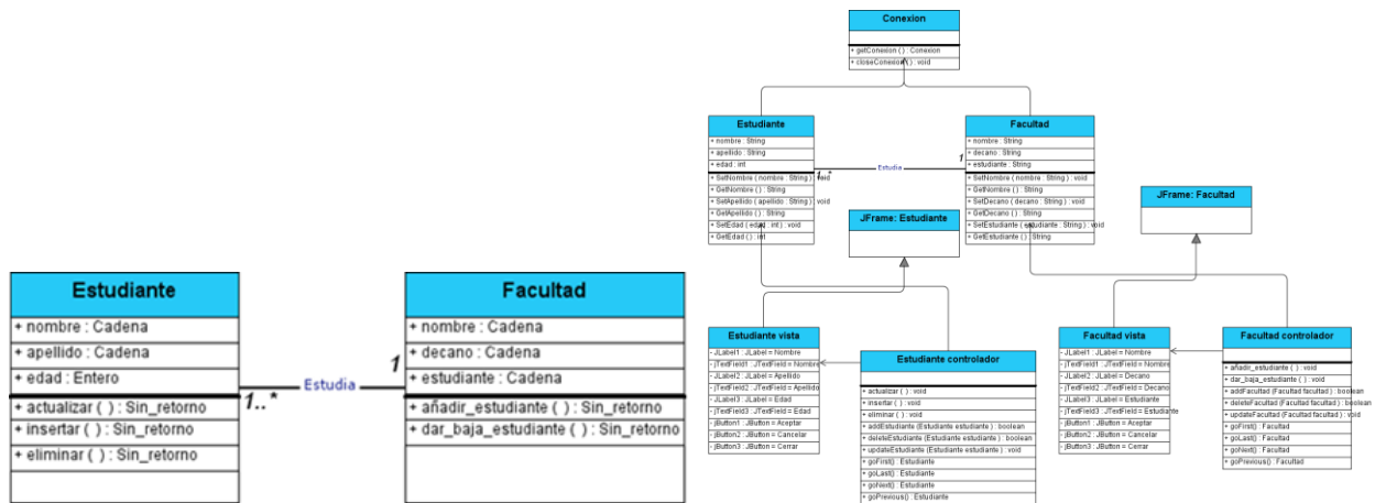
Fig. 4 - Diagrama de clases en PIM y su transformado a PSM.
