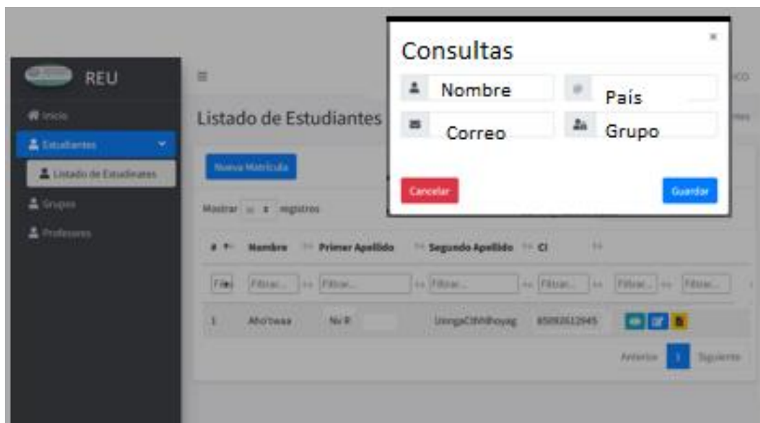
Figura 8. Interfaz «Consulta».
