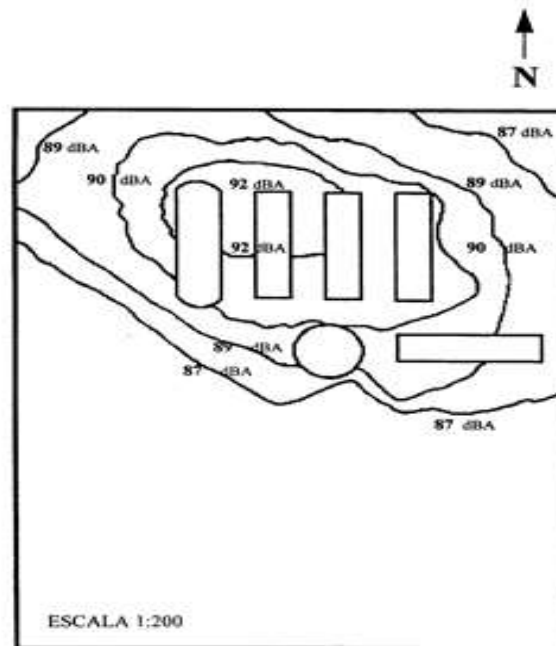
Fig. 3. Mapa de ruido analítico, coplanar. Monocromático, con representación de isolíneas de intensidad sonora.
