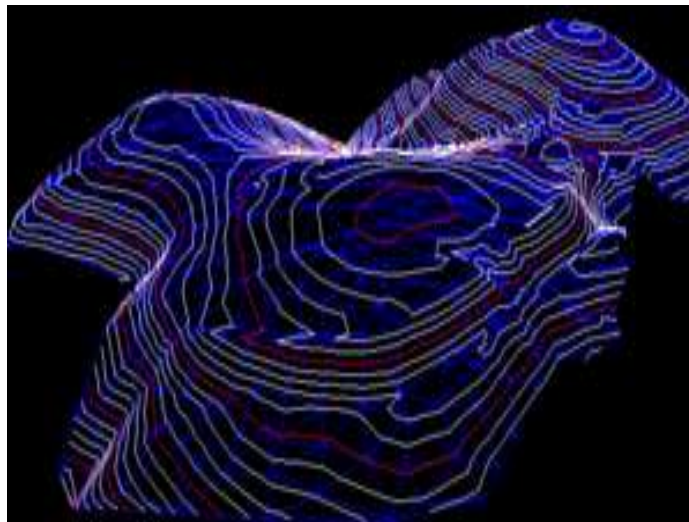
Fig. 4. Mapa de ruido analítico en 3D. Policromático con presentación de posibles isolíneas de intensidad sonora y curvas de nivel topográfico.
