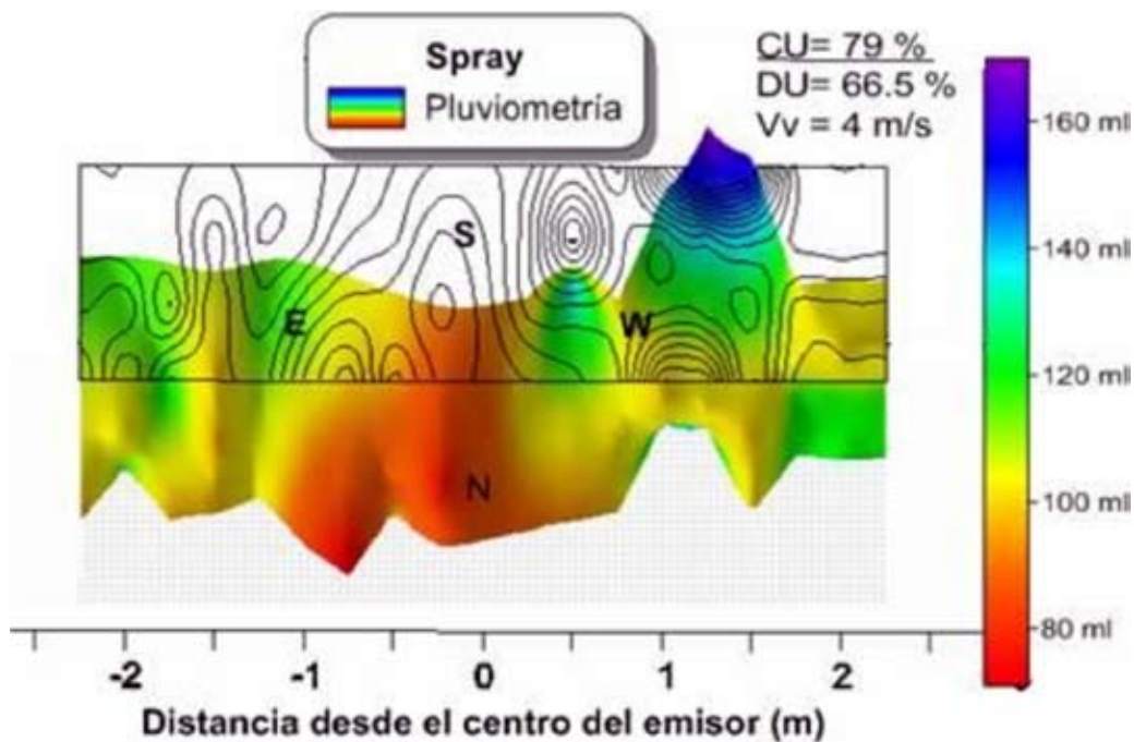
FIGURA 5. Pluviometría tridimensional del emisor espaciado a 2,80 m y a una presión de 160 kPa.
