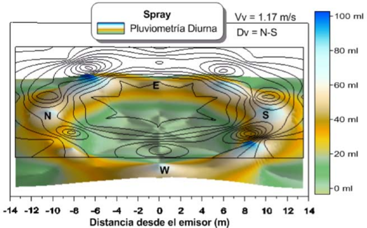
FIGURA 3. Pluviométrica tridimensional a una presión de 200 kPa a 2 m de altura respecto a la superficie del suelo.
