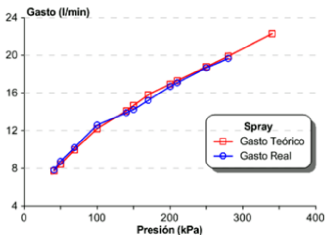
FIGURA 1. Curva del gasto en función de la presión (real y teórico).
