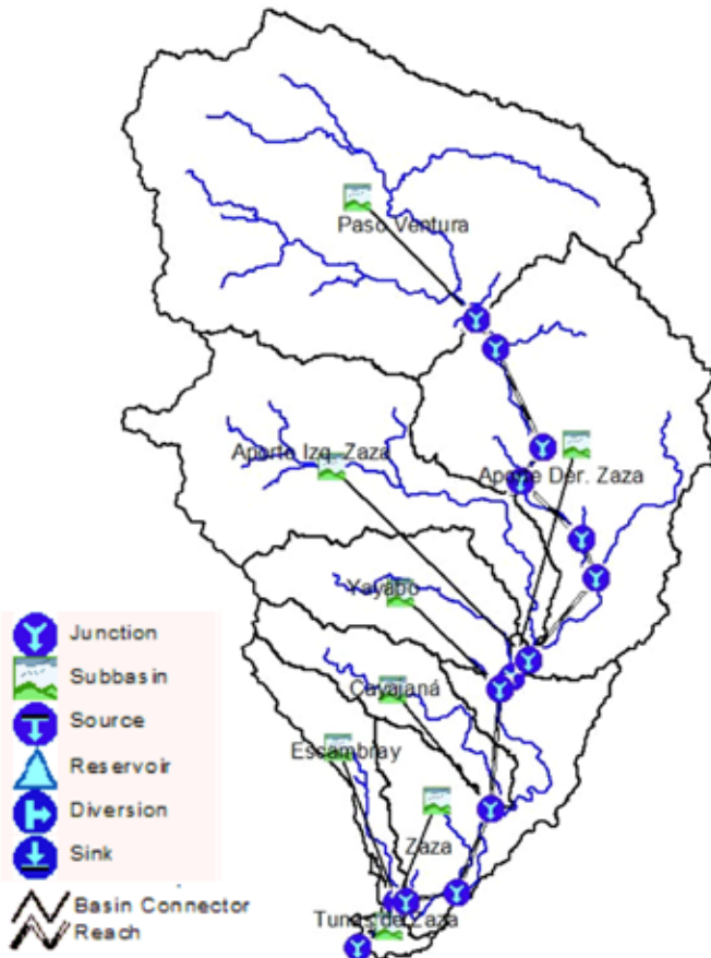
FIGURA 1. Modelo hidrológico conceptual preliminar de Cuenca Zaza a exportar al HEC-HMS.
