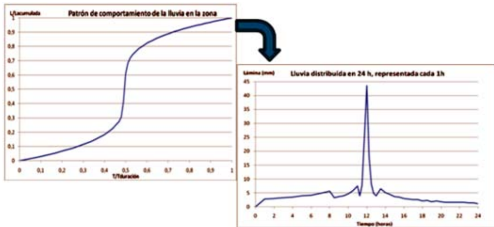
FIGURA 2. Ejemplo del dimensionamiento del patrón de comportamiento de la tormenta tipo III en un hietograma para una lluvia del 1% de probabilidad para una zona en la cuenca del río Zaza.
