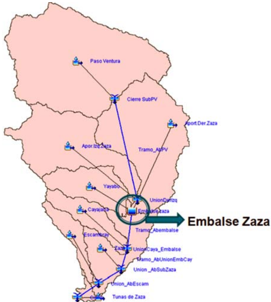
FIGURA 5. Modelo hidrológico conceptual de la cuenca del río Zaza, incluyendo el embalse.
