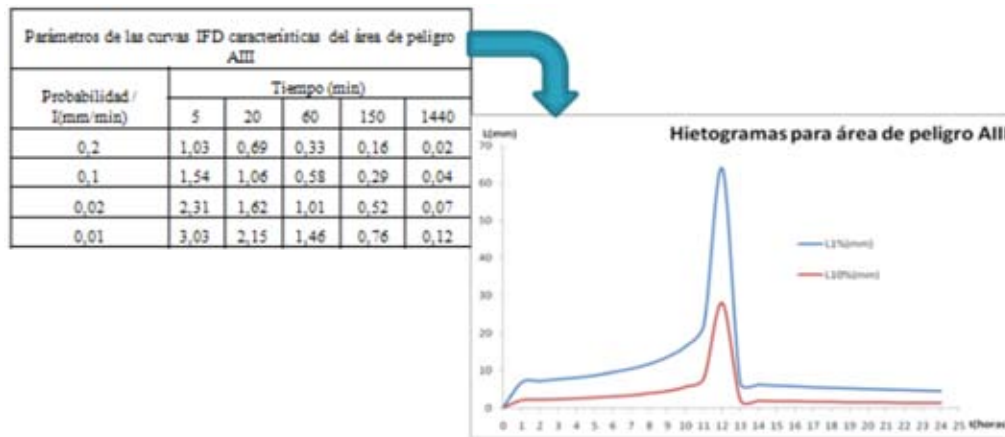
FIGURA 4. Obtención de los hietogramas con duración de 24 horas y probabilidades de 1 y 10% a partir de las curvas IFD obtenidas por Planos et al. (2004), para la cuenca Zaza.
