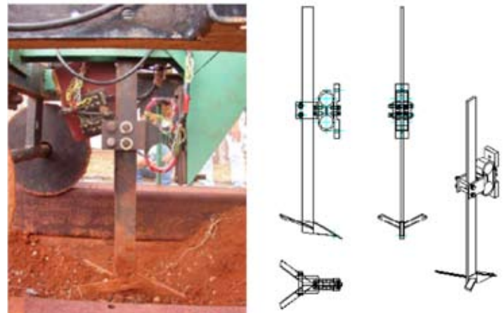
FIGURA 1. Sensor de compactación desarrollado en el CEMA.
