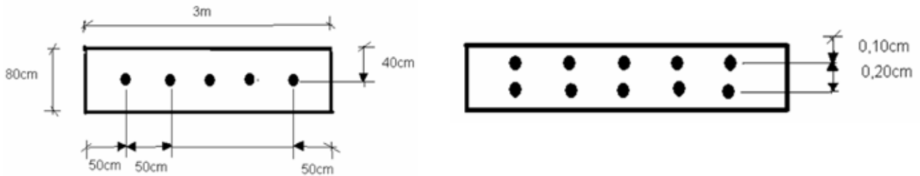
FIGURA 2. Esquema de las zonas de muestreo en el canal de suelos. Vista en planta y lateral.
