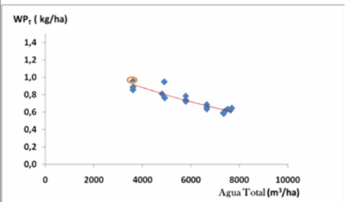
FIGURA 7. Relación entre la productividad del agua total ( WP_T ) y la cantidad de agua total (riego+lluvia) para el sorgo.
