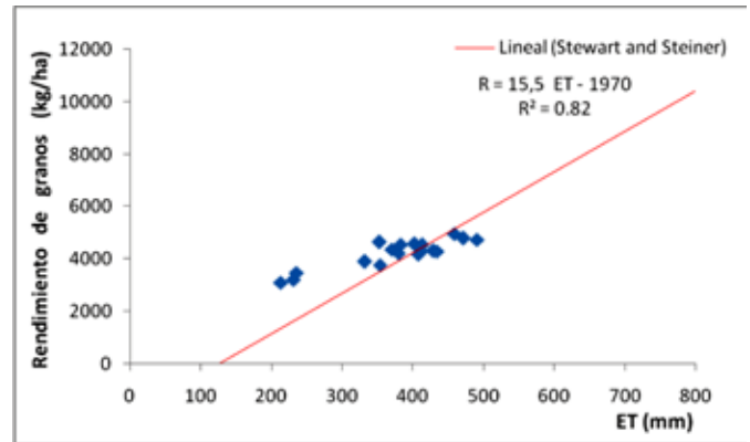
FIGURA 2. Comparación de los resultados de Stewart and Steiner (1990) para el sorgo cultivado en regiones semiáridas con los obtenidos para el sorgo en Cuba.
