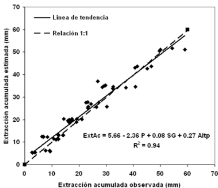
FIGURA 2. Valores estimados y observados para la extracción acumulada del maíz en siembra directa.
