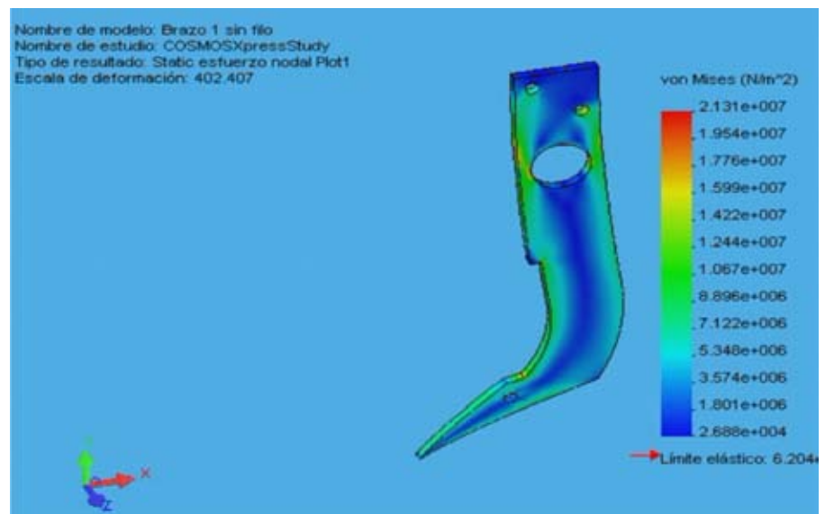
FIGURA 5. Comportamiento del brazo por Elementos Finitos.
