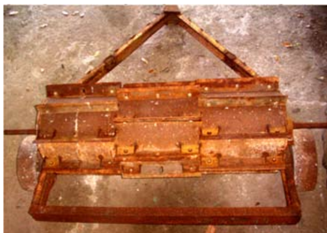
FIGURA 1. Rodillo de cuchillas CEMA 1400 para cobertura vegetal.
