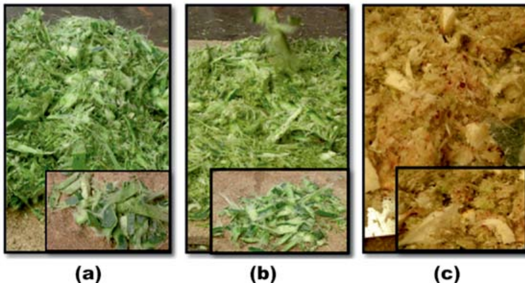
FIGURA 5. Material troceado a 1500 rpm; (a) hojas a 45°; (b) hojas a 90°; (c) piña.
