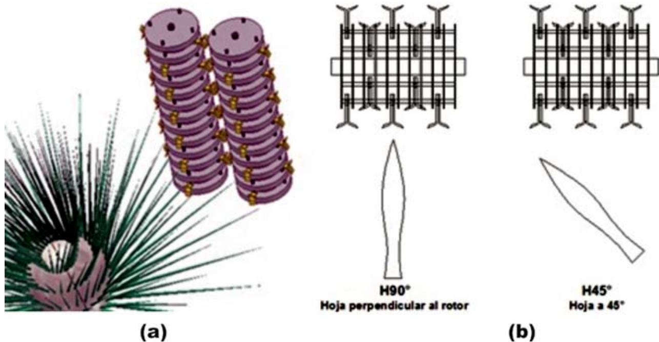
FIGURA 4. Troceado de hoja; (a) esquema propuesto; (b) posiciones extremas de troceado.
