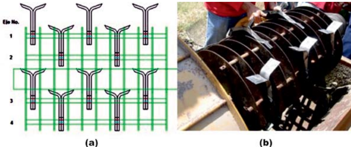
(a) (b) FIGURA 3. Distribución de cuchillas; (a) vista esquemática eje 1 a 4; (b) construidas y acopladas.
