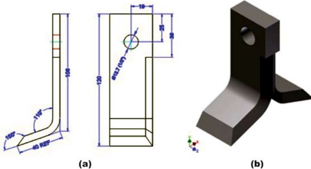
(a) (b) FIGURA 2. Cuchilla; (a) ½”Y” dimensiones; (b)”Y” modelado 3D en Autodesk Inventor 2010.
