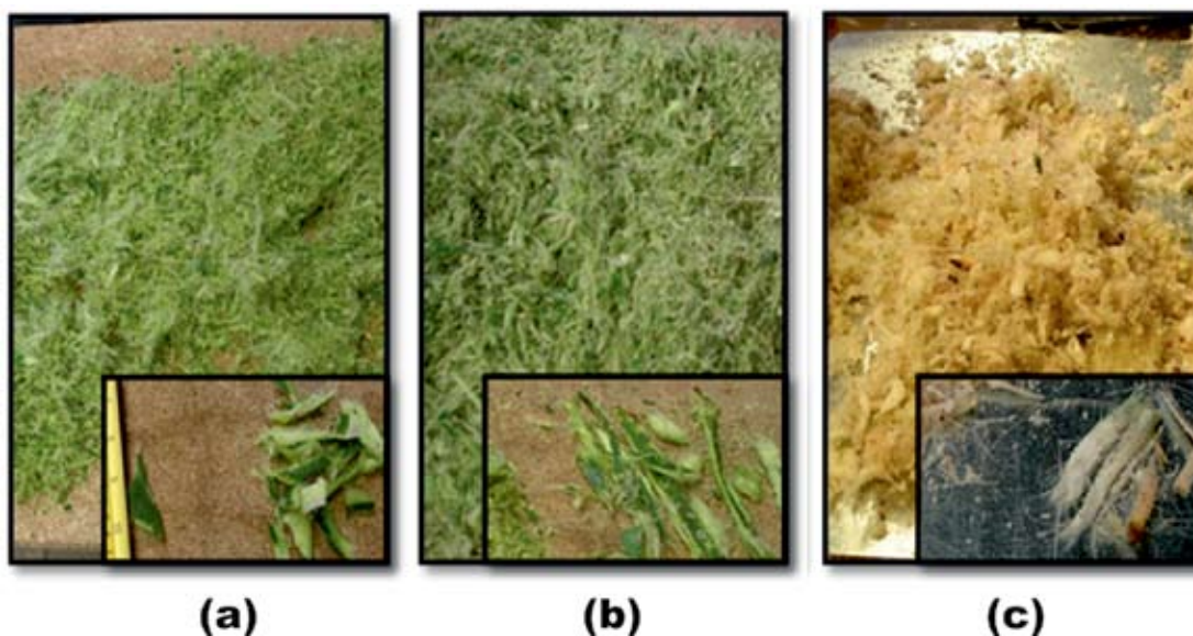
FIGURA 6. Material troceado a 2 000 rpm; (a) hojas a 45 °; (b) hojas a 90°; (c) piña.
