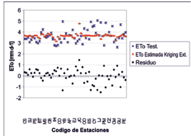
FIGURA 8. Validación cruzada de la ET o con el método de interpolación espacial Kriging ordinario con tendencia externa.
