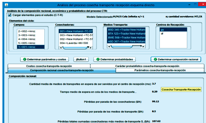
FIGURA 6. Interfaz para la determinación de la composición racional del proceso.
