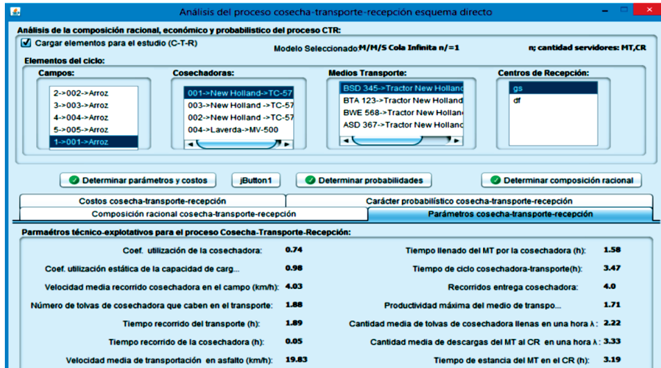
FIGURA 3. Interfaz para los cálculos de los parámetros de explotación.
